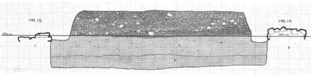
Abb. 29 Kaiseraugst, Im Sager, Parz. 1006. Raum C. Profilaufnahme zwischen MR 19 und MR 15 mit der Benutzungsschicht 5 und dem Gehniveau Schicht 3. M. 1:40.
