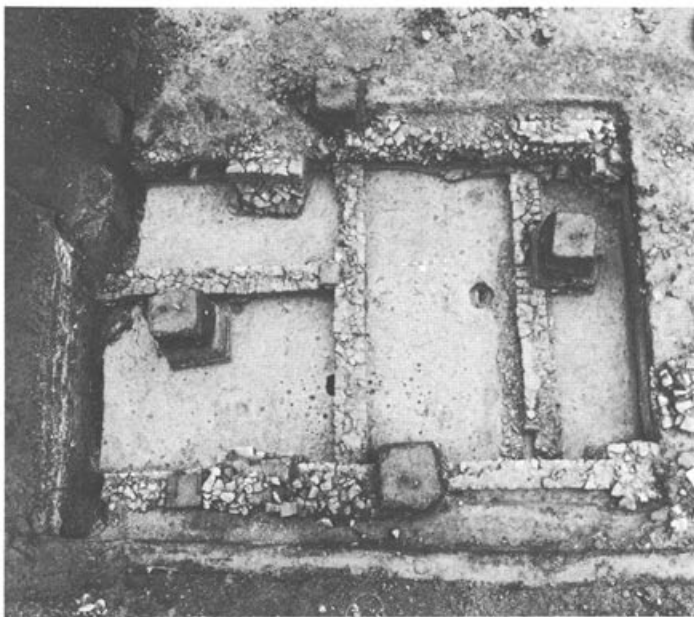
Abb. 1 Augst, H. Moritz, Parz. 1027, Insula 50, Los A. Es zeichnen sich zwischen den Mauerresten der späteren Steinbauten (MR 5,3,4), Spuren von Pfosten und Steinunterlagen für Balken im hellen gewachsenen Lehm ab. Aufsicht vom Kran von Westen.
