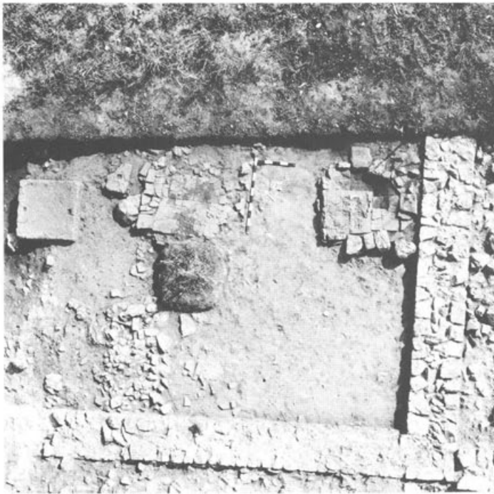
Abb. 20 August, H. Moritz, Parz. 1027. Los D, die Südwestecke der grossen Werkhalle (MR 37, 36) an der Ostrandstrasse gelegen, mit zwei Herdstellen und einer Stützenunterlage, mit der die Halle gegliedert war. Aufsicht von Südwesten.
