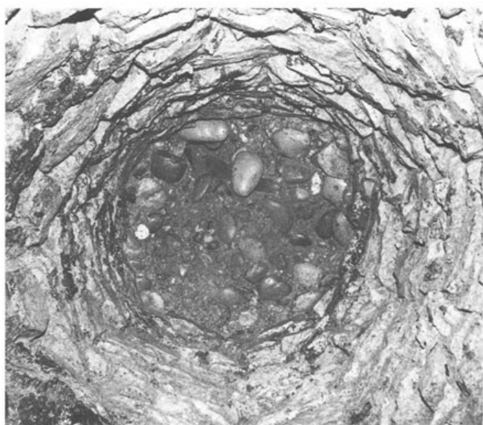
Abb. 21 Kaiseraugst, Auf der Wacht II, Parz. 231. Ostinsula. Brunnenkranz (wie Abb. 20) aus Kalkbruchsteinen ohne Mörtelverband, mit deutlich erkennbarem, anstehendem Kies an der Brunnensohle. Aufsicht.
