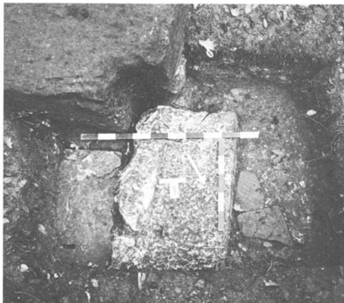
Abb. 31 Augst, Sichelen, Amphitheater, Parz. 1063. Der Torrahmen des Osttores zur Arena mit der Schwelle in situ auf 281,85 m. Aufsicht von Norden.
