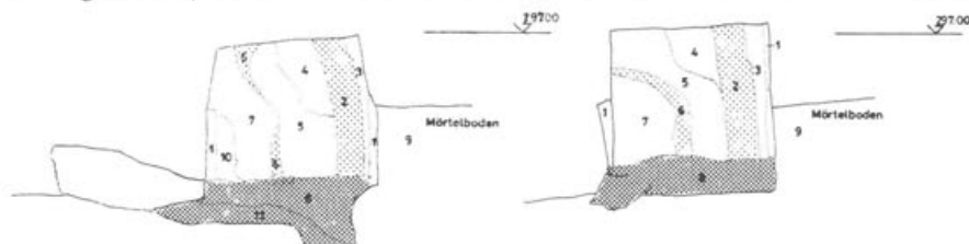
Abb. 10 Augst, H. Moritz, Parz. 1027, Los D, Profilansicht des Lehmstampfkerns mit Schichtenaufbau MR 90 und MR 72.
