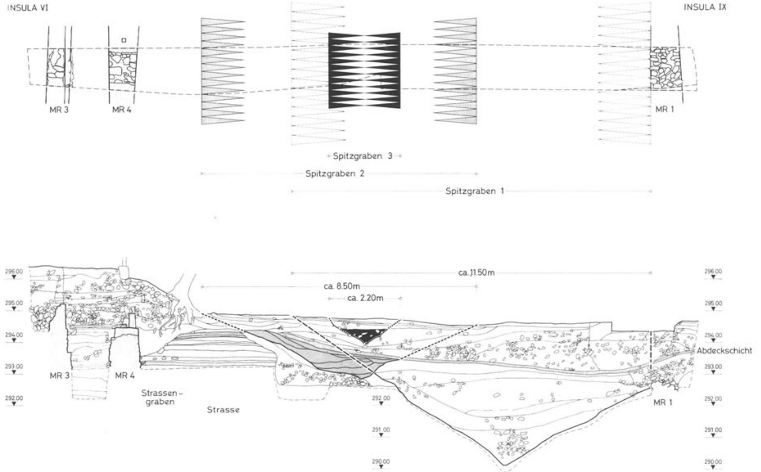
Abb. 38 Augst, FTS-Projekt, Parz. 435/654, Insula 6/9. Schichtenprofil mit Südporticus, Insula 6 (MR 3, 4). Halsgrabenstrasse mit Nordstrassengraben. Spitzgraben 1 und 2 sowie Hausmauer (MR 1), Insula 9, überlagert von Abdeckschicht (schraffiert). Zuoberst Spitzgraben 3. Ansicht von Westen.
