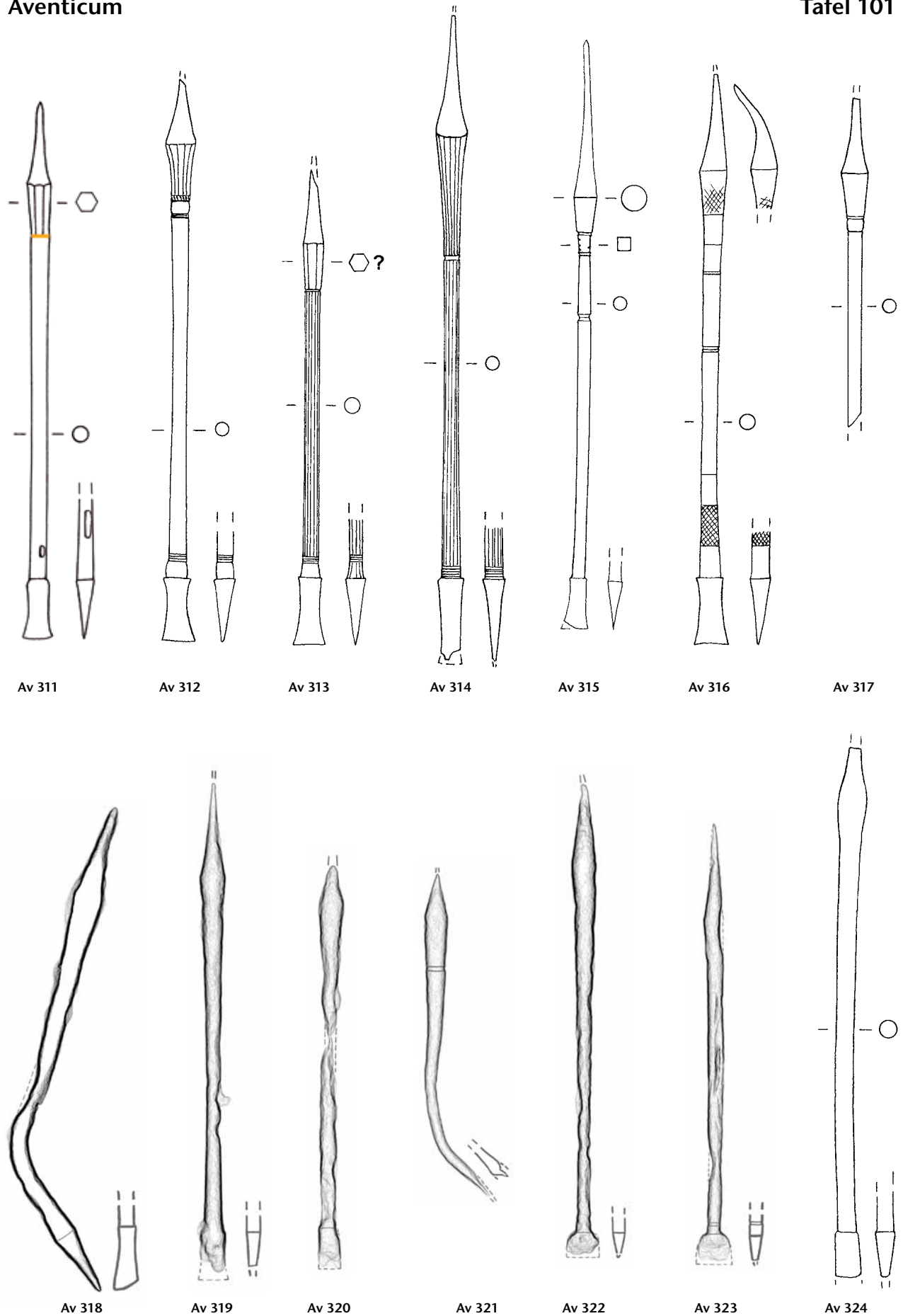
Tafel 101: Aventicum. Formgruppe H 47: Av 311–Av 324. Eisen. M. 3:4.
