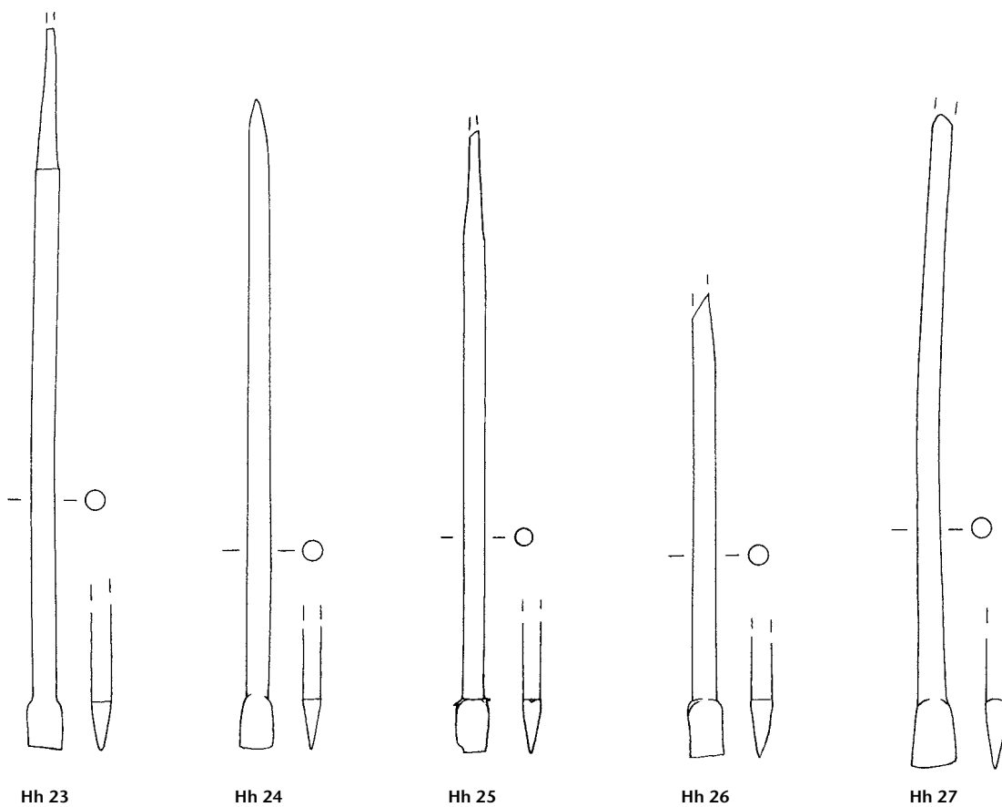
Tafel 174: Hofheim/D. Formgruppe C 23 (Fortsetzung): Hh 17-Hh 27. Eisen. M. 3:4.
