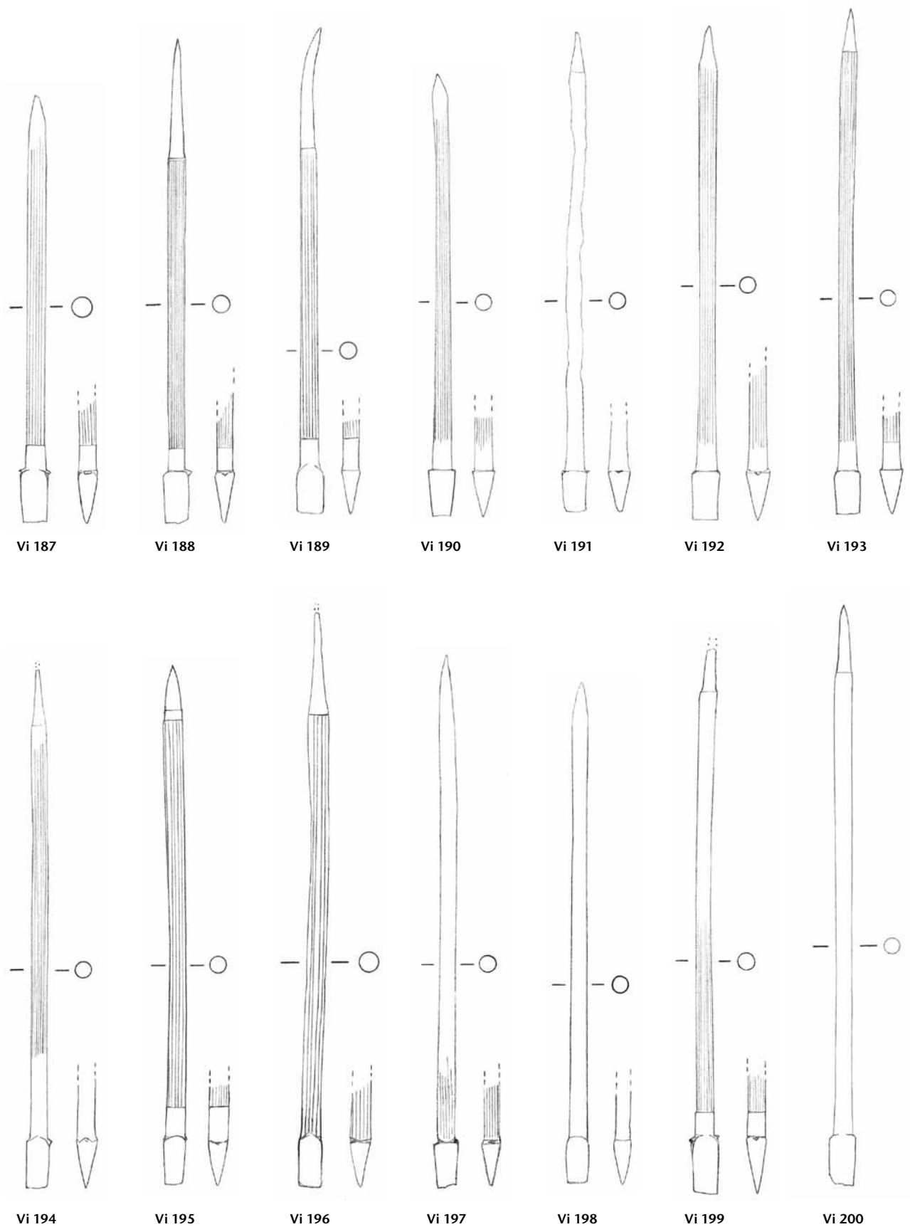
Tafel 133: Vindonissa. Ähnlich Formgruppe C 23: Vi 187-Vi 200. Eisen. M. 3:4.
