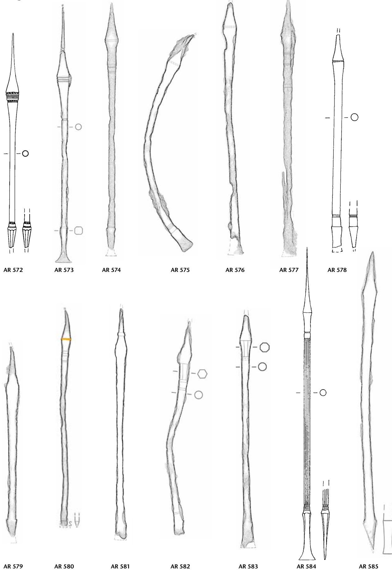
Tafel 37: Augusta Raurica. Formgruppe H 47: AR 572–AR 585. Eisen. M. 3:4.
