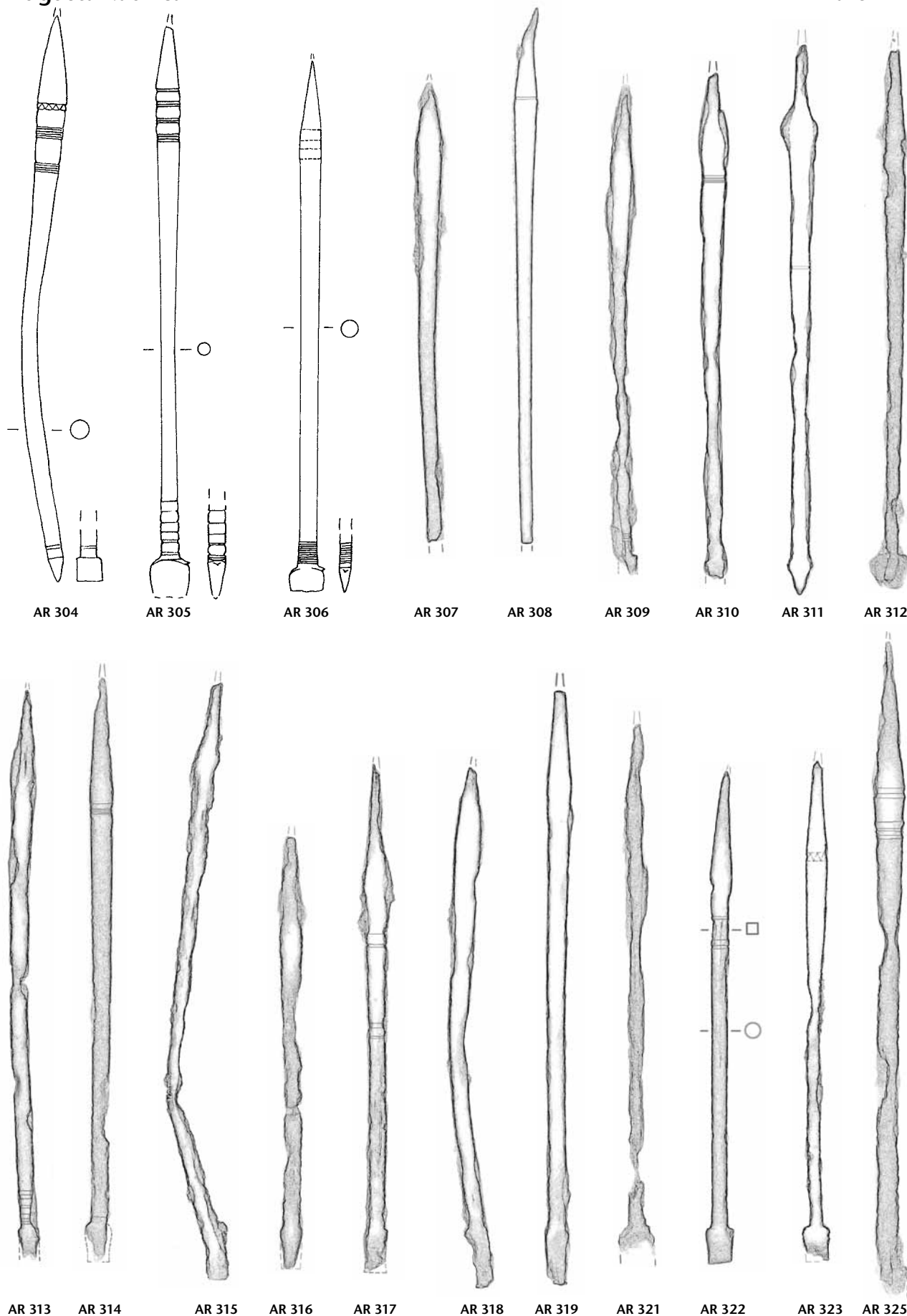
Tafel 21: Augusta Raurica. Formgruppe H 34 (Fortsetzung): AR 304–AR 325. Eisen. M. 3:4.
