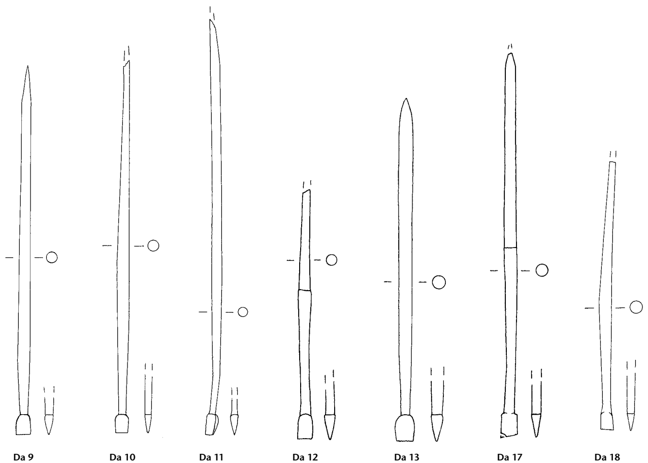
Tafel 165: Dangstetten/D. Formgruppe A 10: Da 1-Da 18. Eisen (Da 5 Buntmetall). M. 3:4.
