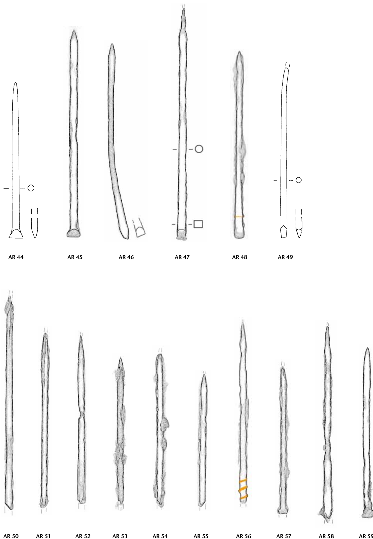
Tafel 4: Augusta Raurica. Formgruppe B 16: AR 44–AR 49. Formgruppe C 22: AR 50–AR 59. Eisen. M. 3:4.
