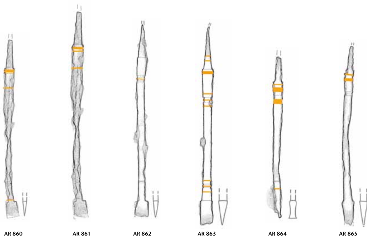
Tafel 57: Augusta Raurica. Formgruppe Q 71: AR 852–AR 865. Eisen. M. 3:4.
