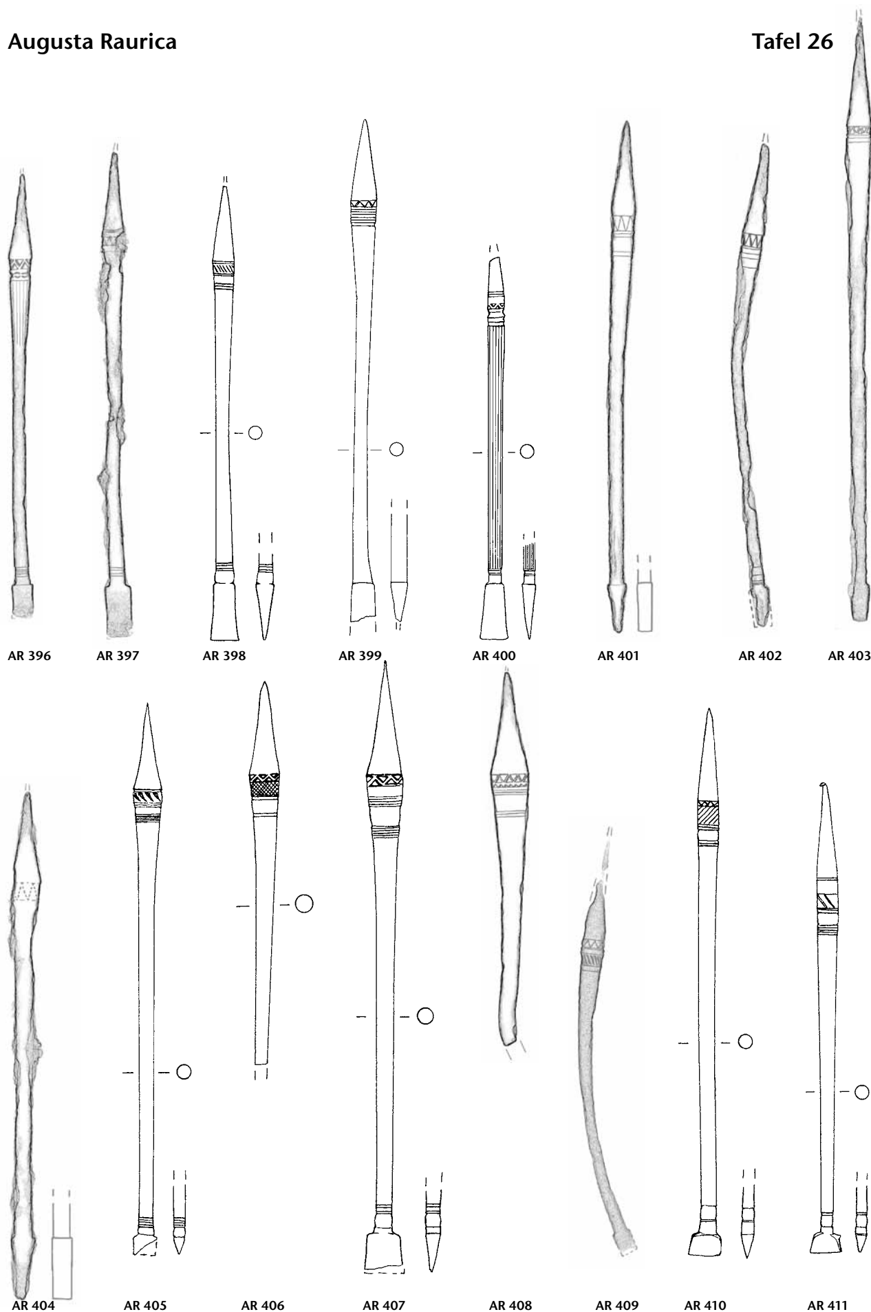
Tafel 26: Augusta Raurica. Formgruppe H 35 (Fortsetzung): AR 396–AR 411. Eisen. M. 3:4.
