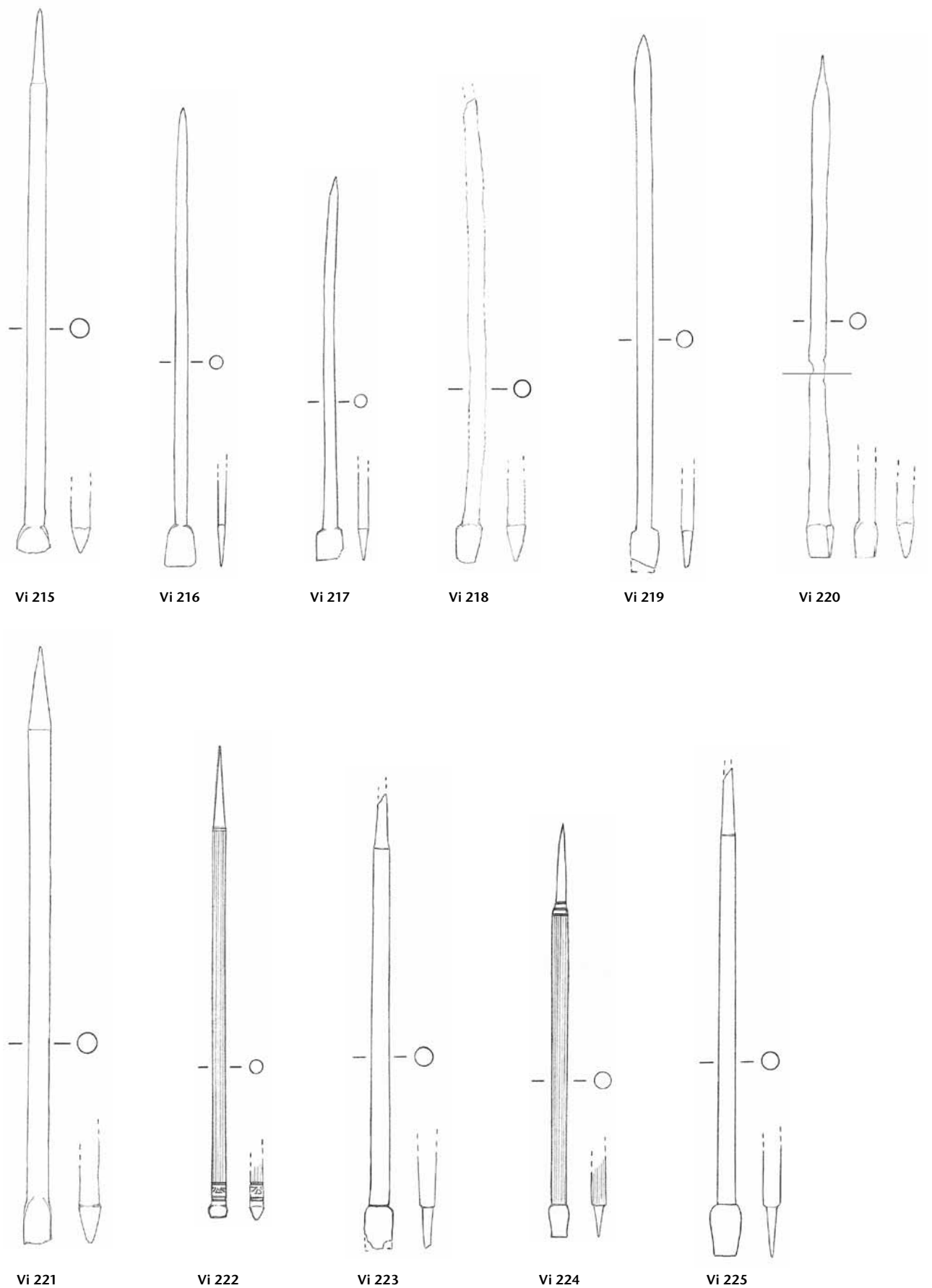
Tafel 135: Vindonissa. Ähnlich Formgruppe C 23 (Fortsetzung): Vi 215–Vi 225. Eisen. M. 3:4.
