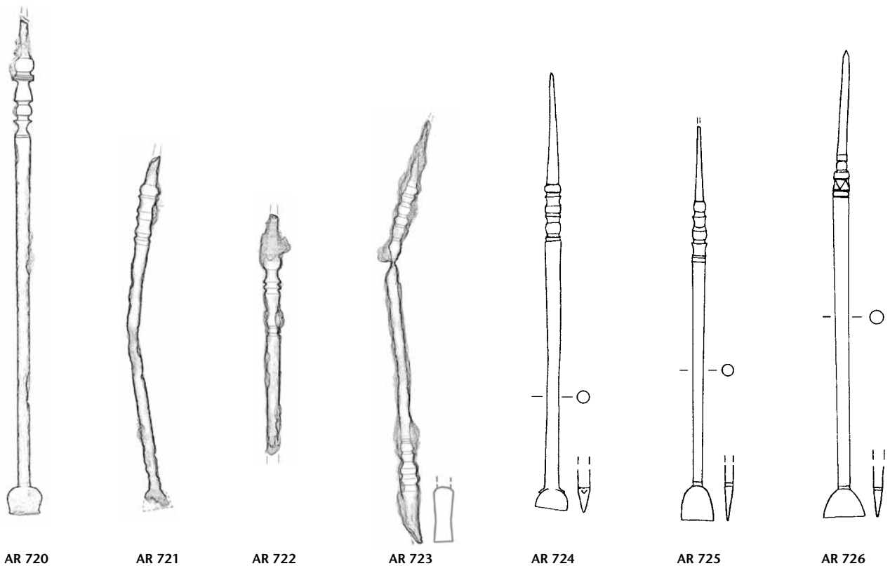
Tafel 47: Augusta Raurica. Formgruppe P 54: AR 720–AR 726. Eisen. M. 3:4.
