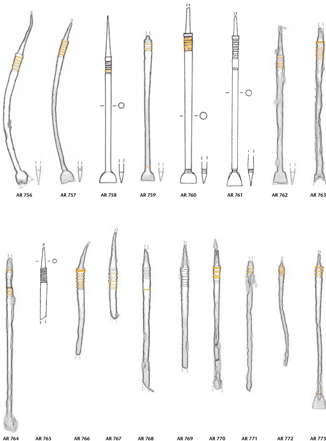
Tafel 50: Augusta Raurica. Formgruppe P 56 (Fortsetzung): AR 756–AR 773. Eisen. M. 3:4.
