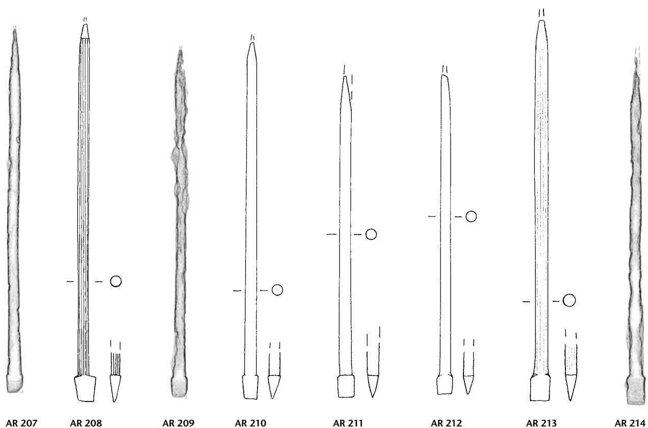
Tafel 14: Augusta Raurica, Formgruppe C 24 (Fortsetzung): AR 198–AR 214. Eisen. M. 3:4.
