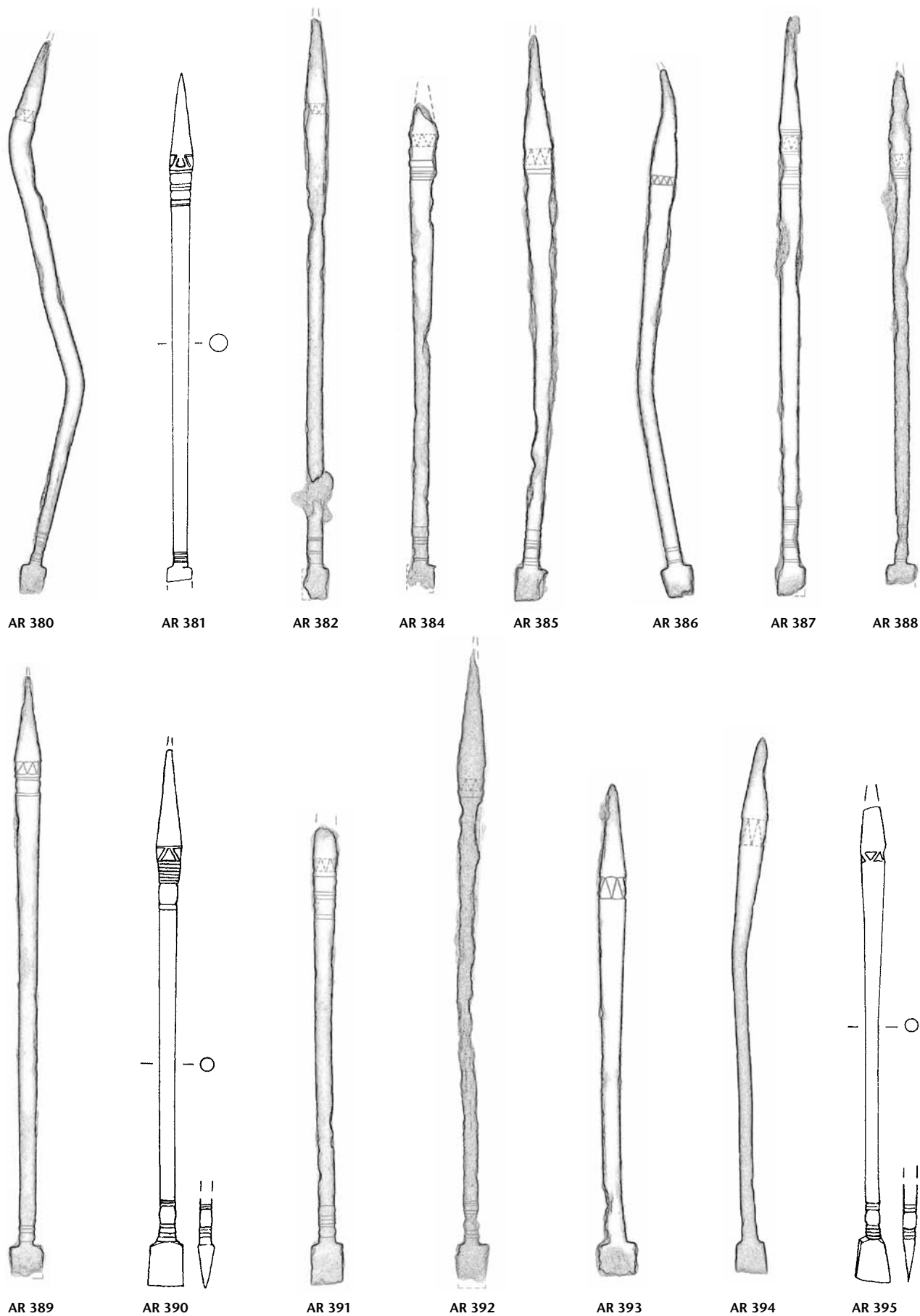
Tafel 25: Augusta Raurica. Formgruppe H 35 (Fortsetzung): AR 380–AR 395. Eisen. M. 3:4.
