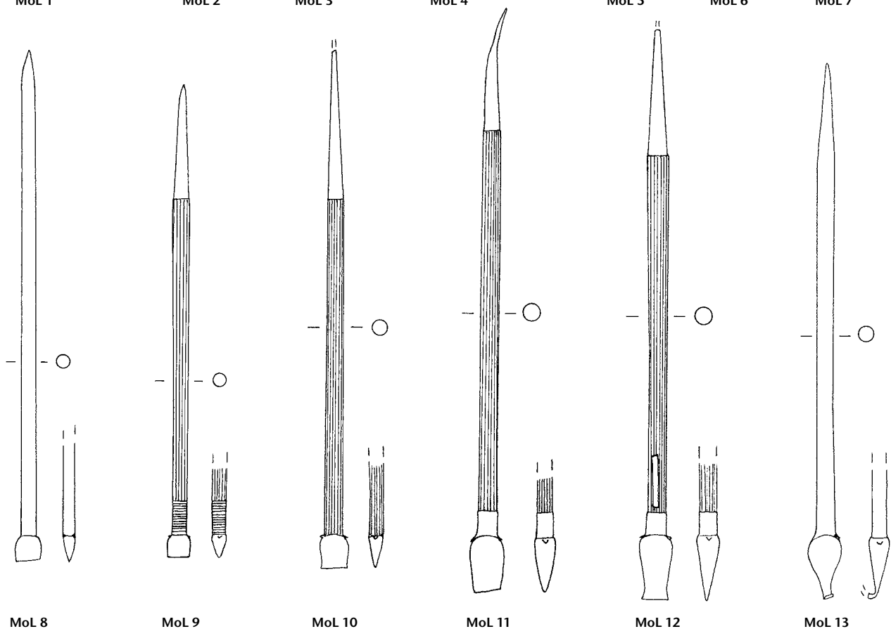
Tafel 185: Museum of London, London/GB. Formgruppe A 10: MoL 1 . Formgruppe B 15: MoL 2–MoL 4 . Formgruppe B 16: MoL 5–MoL 7 . Formgruppe C 23: MoL 8–MoL 13 . Eisen ( MoL 1 , MoL 2 Buntmetall). M. 3:4.
