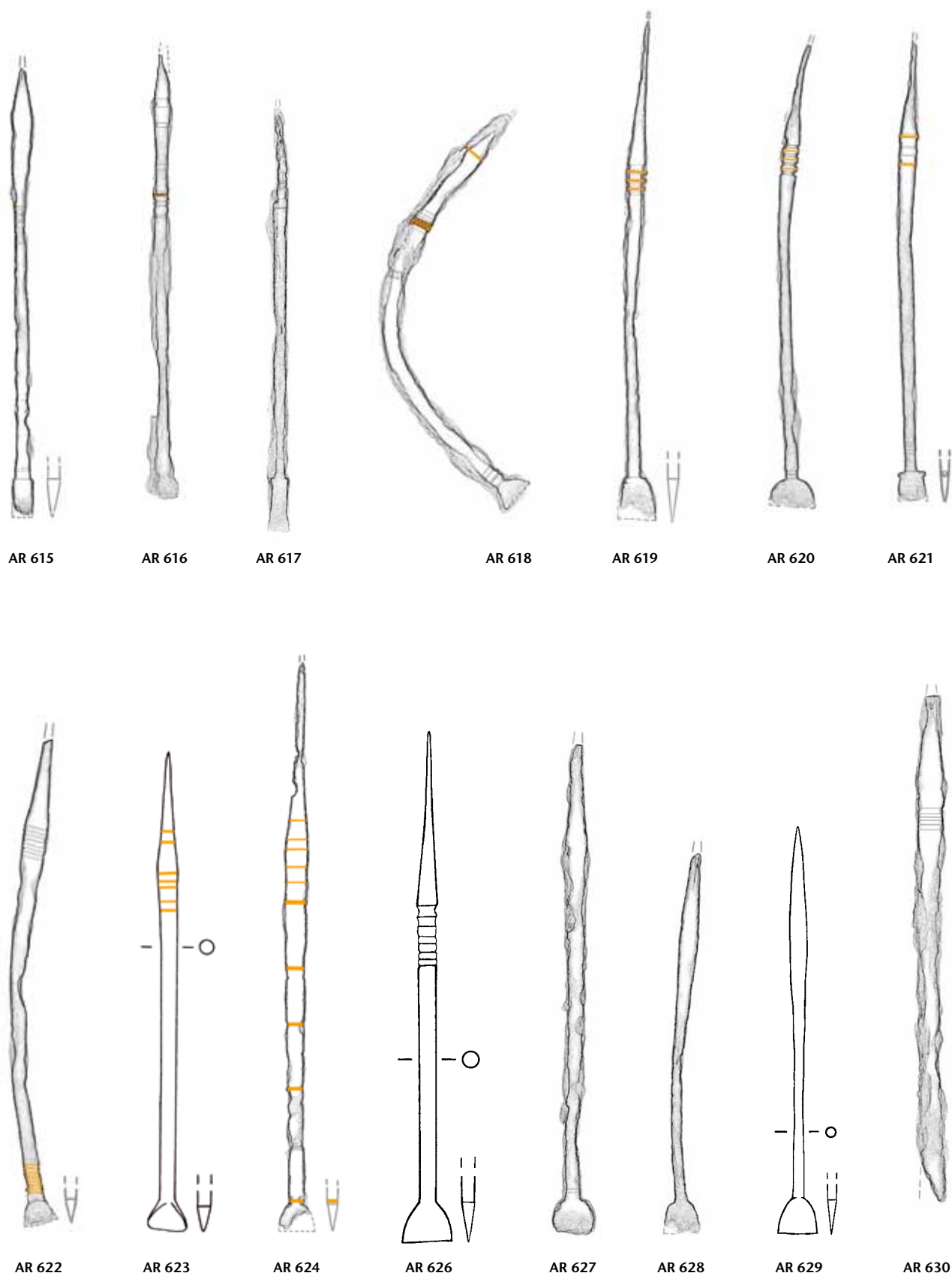
Tafel 40: Augusta Raurica. Formgruppe P 51 (Fortsetzung): AR 615–AR 630. Eisen. M. 3:4.
