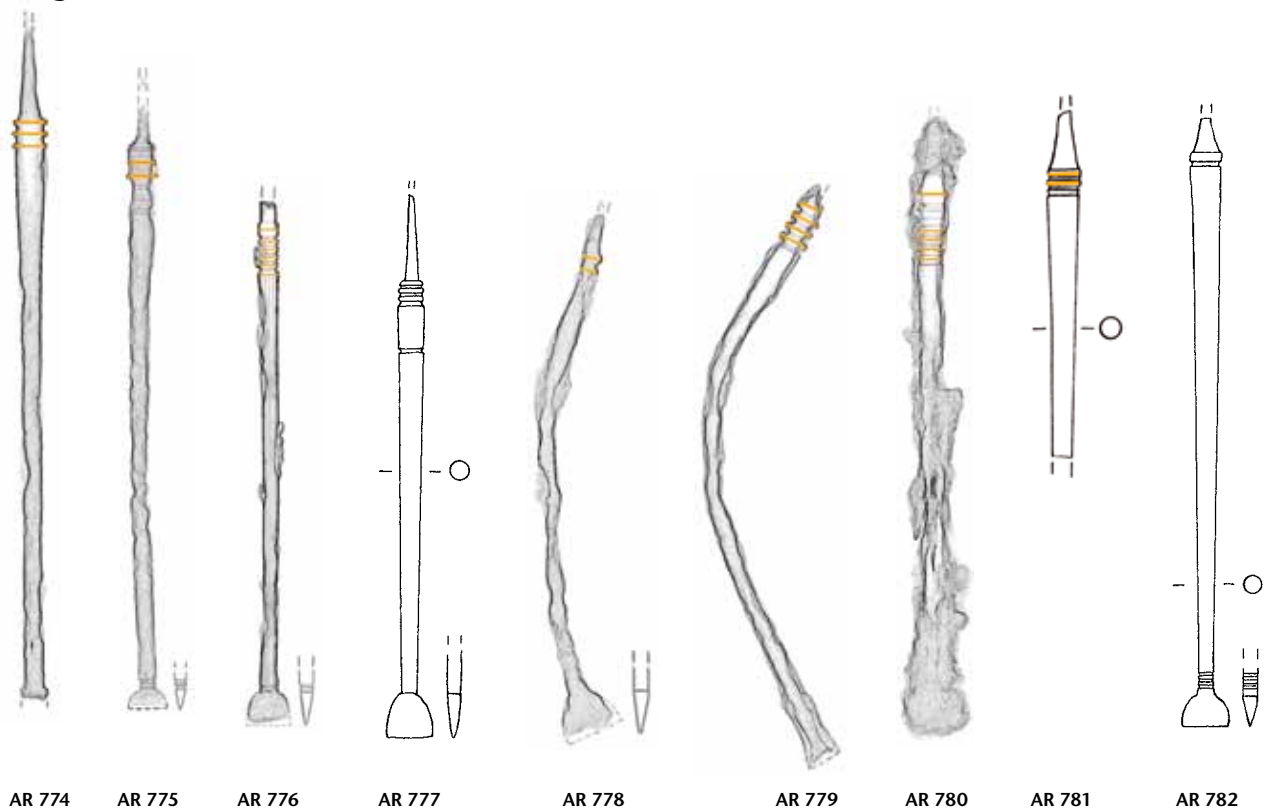
Tafel 51: Augusta Raurica. Formgruppe P 56 (Fortsetzung): AR 774–AR 782. Eisen. M. 3:4.
