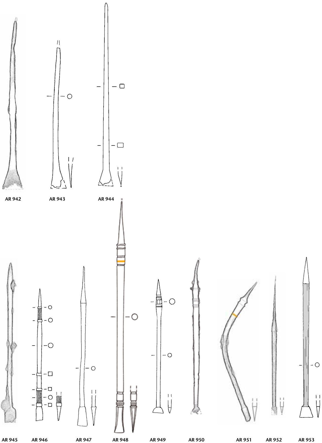
Tafel 64: Augusta Raurica. Formgruppe W 95: AR 942–AR 944. Keiner Formgruppe zugewiesene Einzelfunde: AR 945–AR 953. Eisen (AR 946 Buntmetall). M. 3:4.
