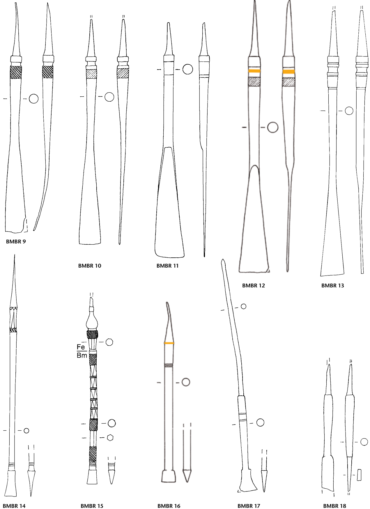
Tafel 194: British Museum, Department of Prehistory and Early Europe, London/GB. Formgruppe H 32: BMBR 9–BMBR 13 . Formgruppe H 35: BMBR 14 . Formgruppe Q 68: BMBR 15 . Formgruppe Q 70: BMBR 16 . Formgruppe V 92: BMBR 17 . Keiner Formgruppe zuweisbares Stück: BMBR 18 . Eisen ( BMBR 15 Messing bzw. Buntmetall). M. 3:4.
