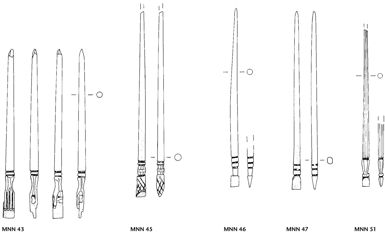
Tafel 203: Neapel/I und Pompeji/I. Beinspindeln oder Beingriffel (Form 1 nach Gostenčnik 1995 und 2005)? (Fortsetzung): MNN 28–MNN 38. Haarnadeln aus Bein: MNN 43–MNN 51. M. 3:4.
