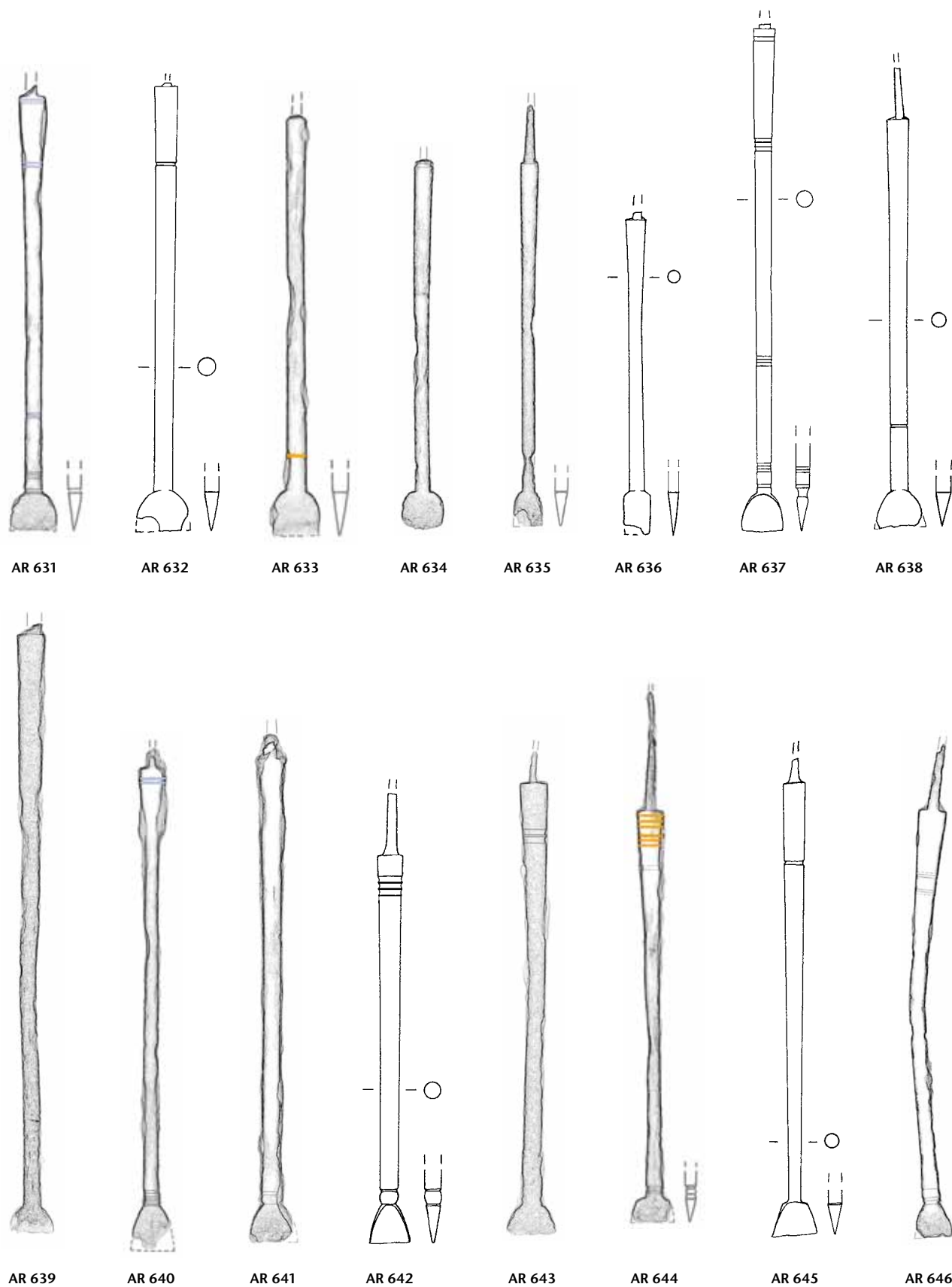
Tafel 41: Augusta Raurica. Formgruppe P 52: AR 631–AR 646. Eisen. M. 3:4.
