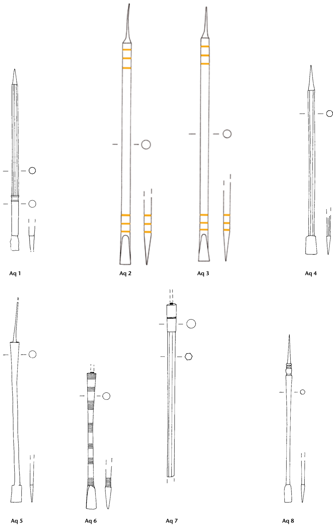
Tafel 196: Aquileia/I – Altfunde. Formgruppe A 10: Aq 1 . Formgruppe C 22: Aq 2 , Aq 3 . Formgruppe C 24: Aq 4 . Formgruppe P 52: Aq 5 – Aq 7 . Formgruppe P 55: Aq 8 . Eisen ( Aq 4 , Aq 6 – Aq 8 Buntmetall). M. 3:4.
