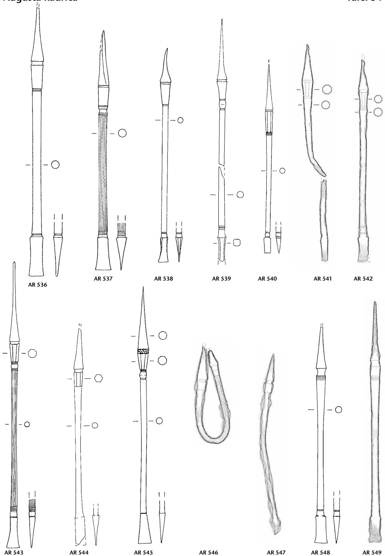
Tafel 34: Augusta Raurica. Formgruppe H 43 (Fortsetzung): AR 536–AR 549. Eisen (AR 536 Bein). M. 3:4.
