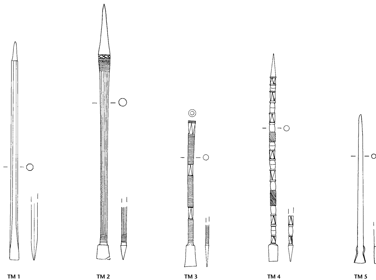
Tafel 204: Toulouse/F (TM). Formgruppe B 15: TM 1 . Formgruppe H 35: TM 2 . Formgruppe P 52: TM 3 . Formgruppe P 57: TM 4 . Keiner Formgruppe zugewiesen: TM 5 . Eisen ( TM 3 , TM 4 Buntmetall). M. 3:4.
