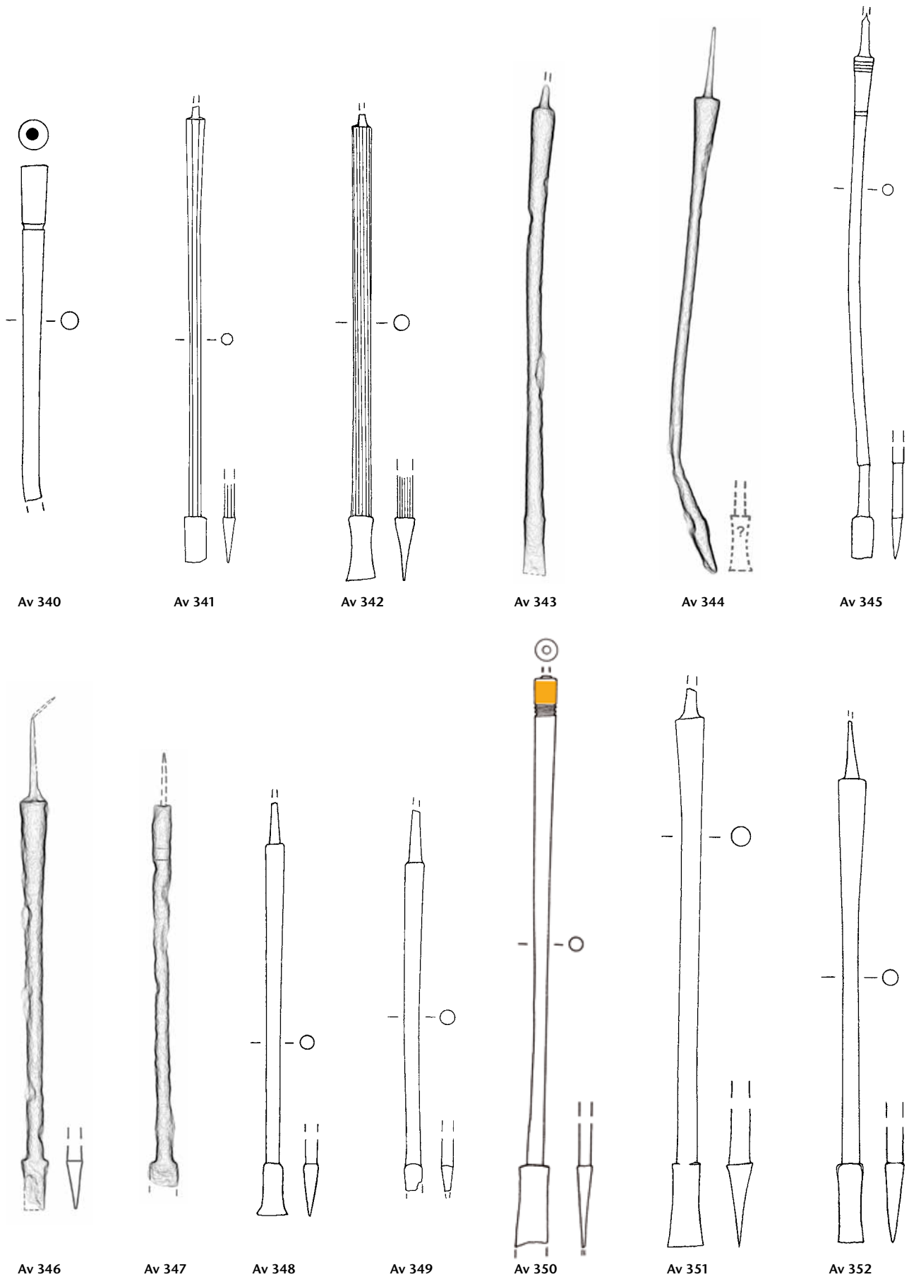
Tafel 103: Aventicum. Formgruppe P 52 (Fortsetzung): Av 340–Av 352. Eisen (Av 340 Buntmetall). M. 3:4.
