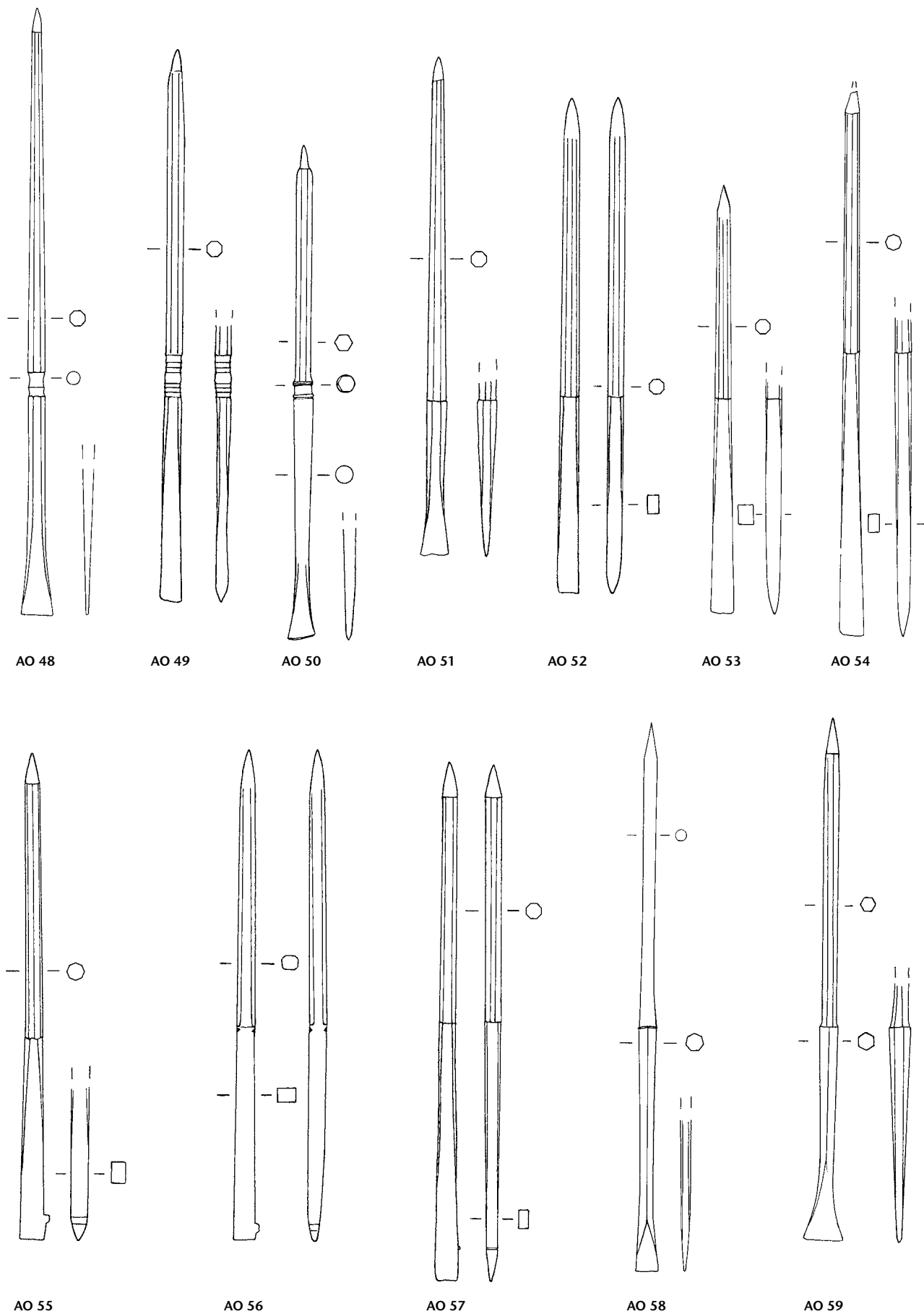
Tafel 170: Augsburg-Oberhausen/D. Formgruppe A 12 (Fortsetzung): AO 48–AO 59. Eisen. M. 3:4.
