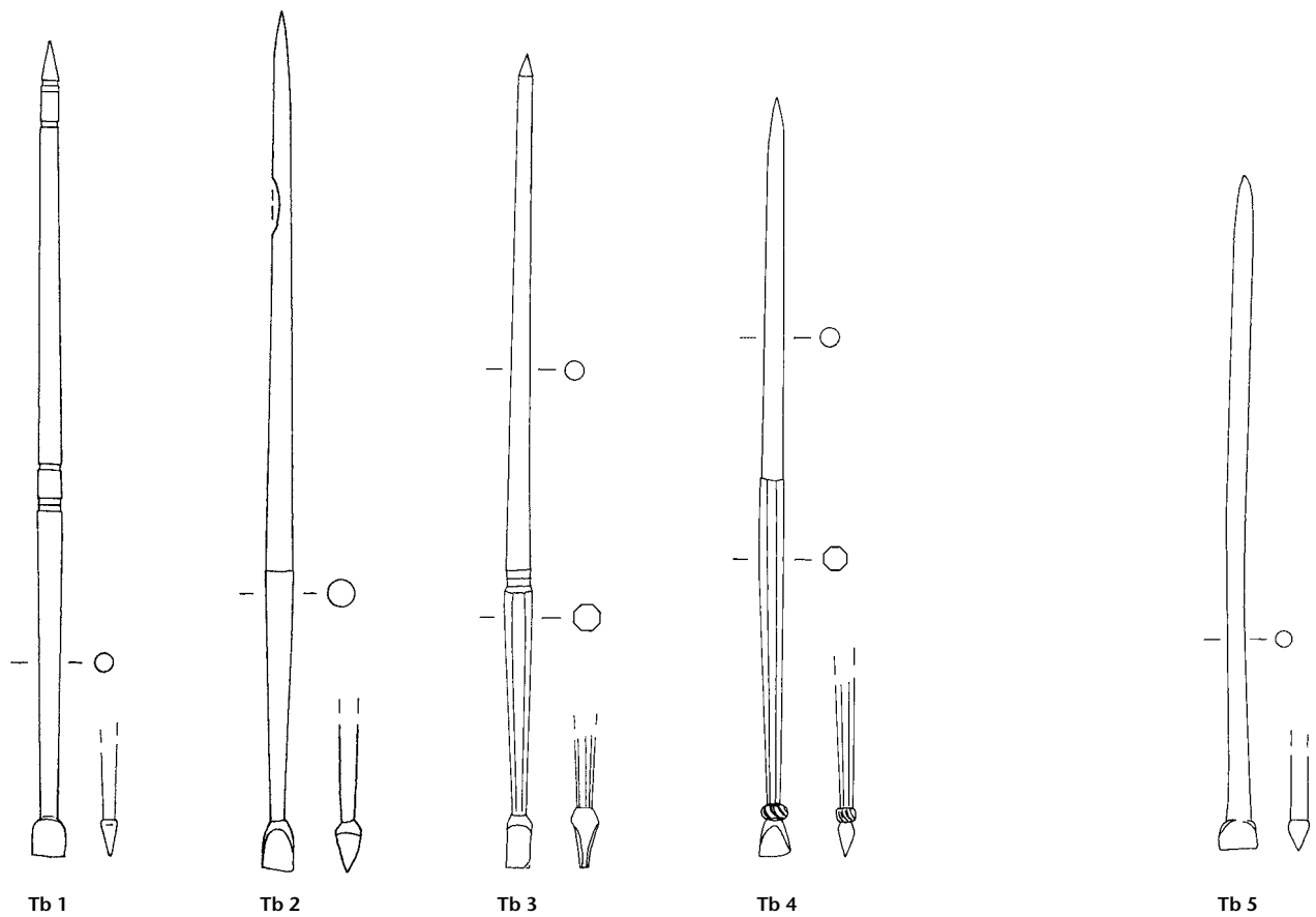
Tafel 182: Titelberg/L – Hortfund. Formgruppe A 10: Tb 1–Tb 4 . Formgruppe C 23: Tb 5 . Eisen. M. 3:4.
