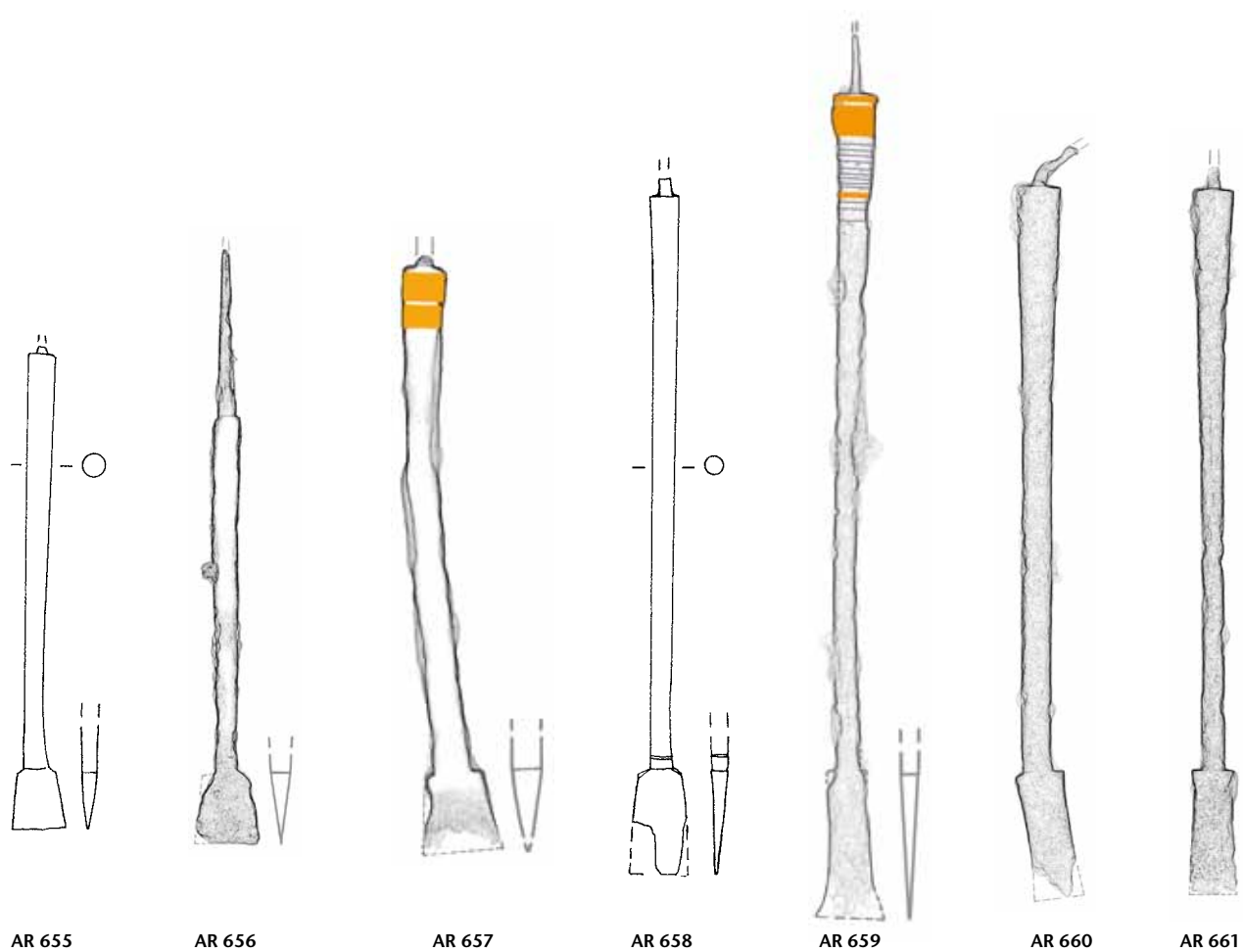
Tafel 42: Augusta Raurica. Formgruppe P 52 (Fortsetzung): AR 647–AR 661. Eisen. M. 3:4.
