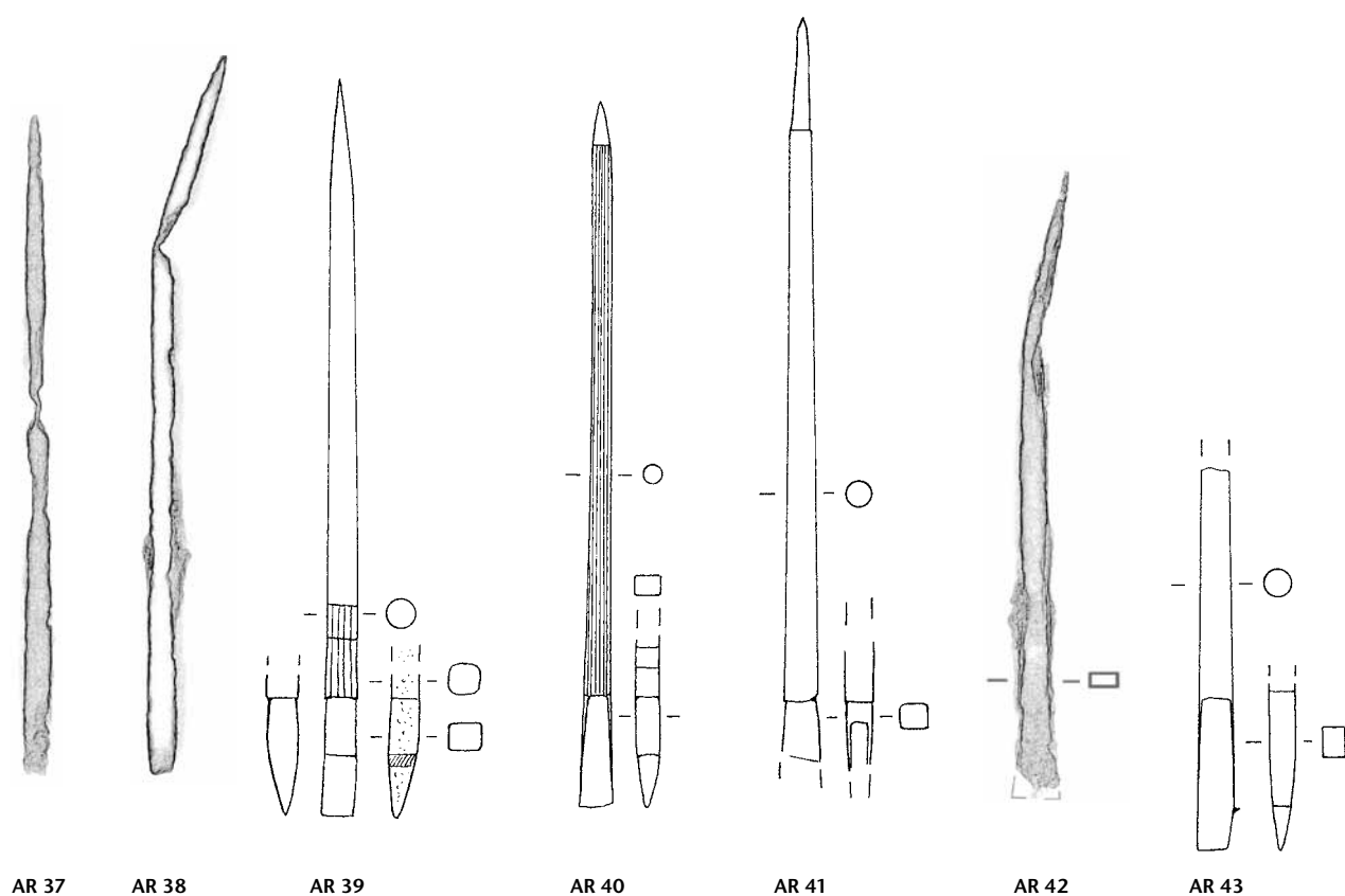
Tafel 3: Augusta Raurica, Formgruppe B 15: AR 28–AR 43. Eisen, M. 3:4.
