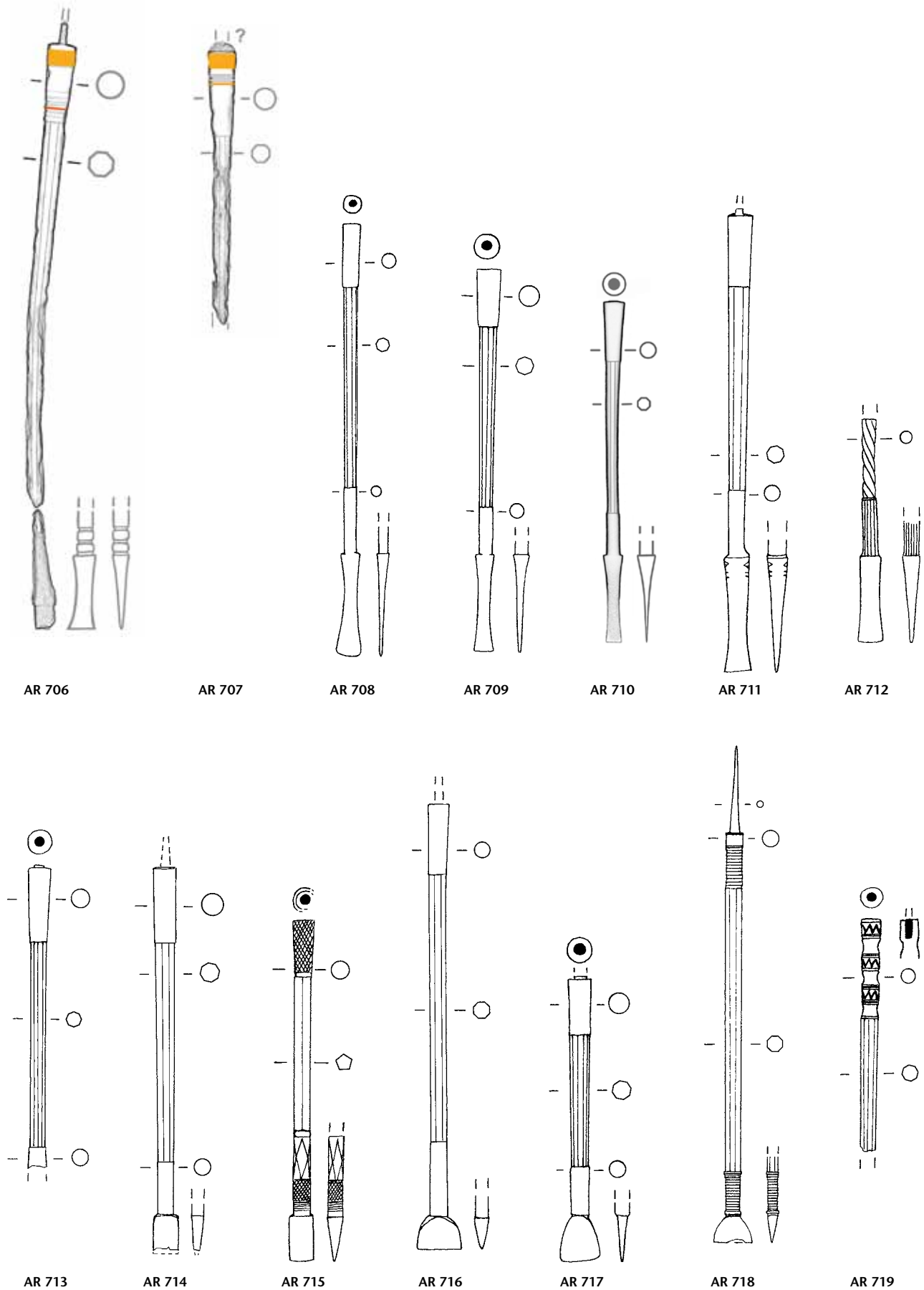
Tafel 46: Augusta Raurica. Formgruppe P 53: AR 706–AR 719. Buntmetall (AR 706, AR 707, AR 711, AR 714, AR 716, AR 718 Eisen). M. 3:4.
