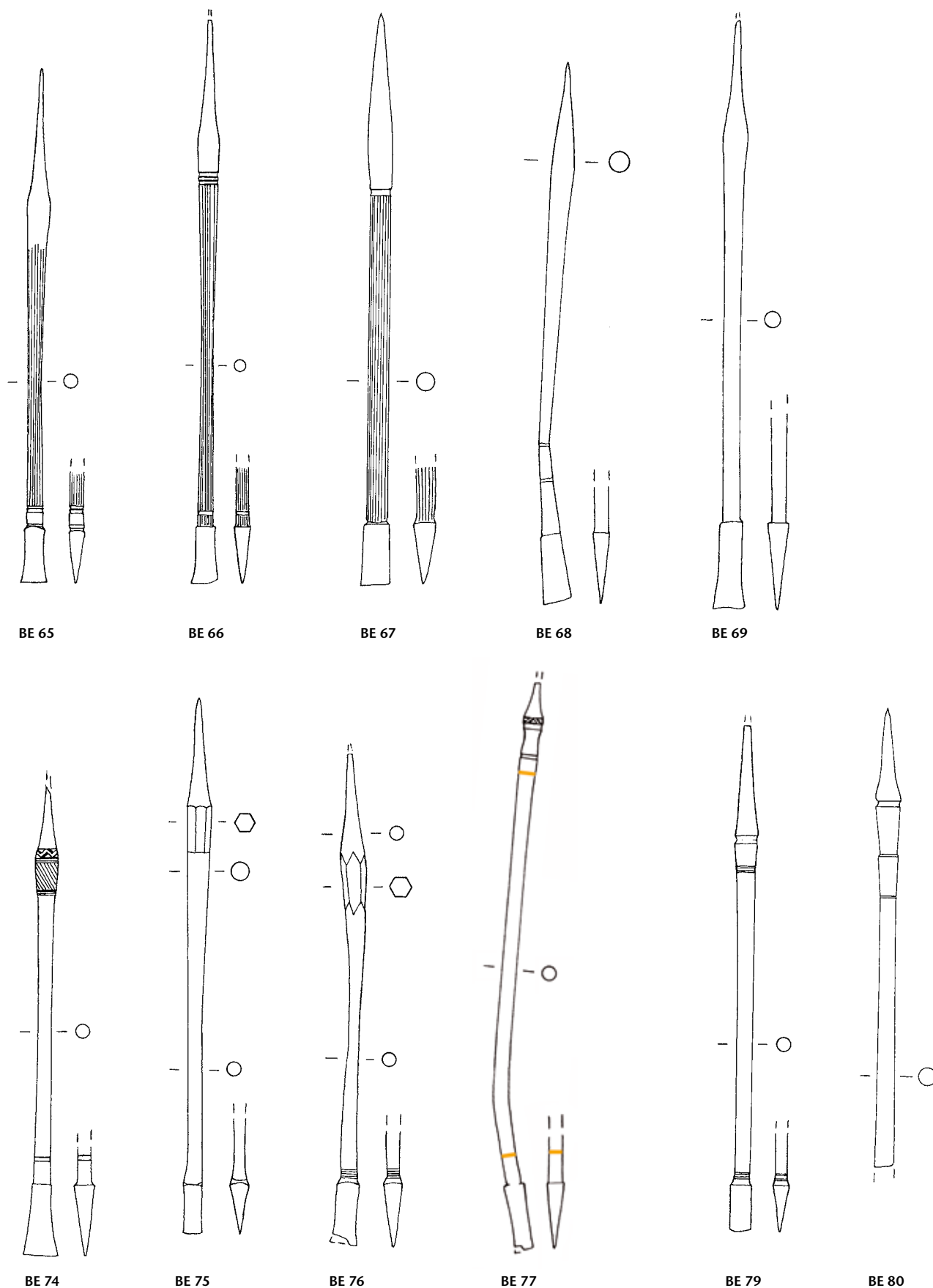
Tafel 160: Bern-Engelhalbinsel. Formgruppe H 34 (Fortsetzung): BE 65–BE 69. Formgruppe H 35: BE 74–BE 77. Formgruppe H 43: BE 79, BE 80. Eisen. M. 3:4.
