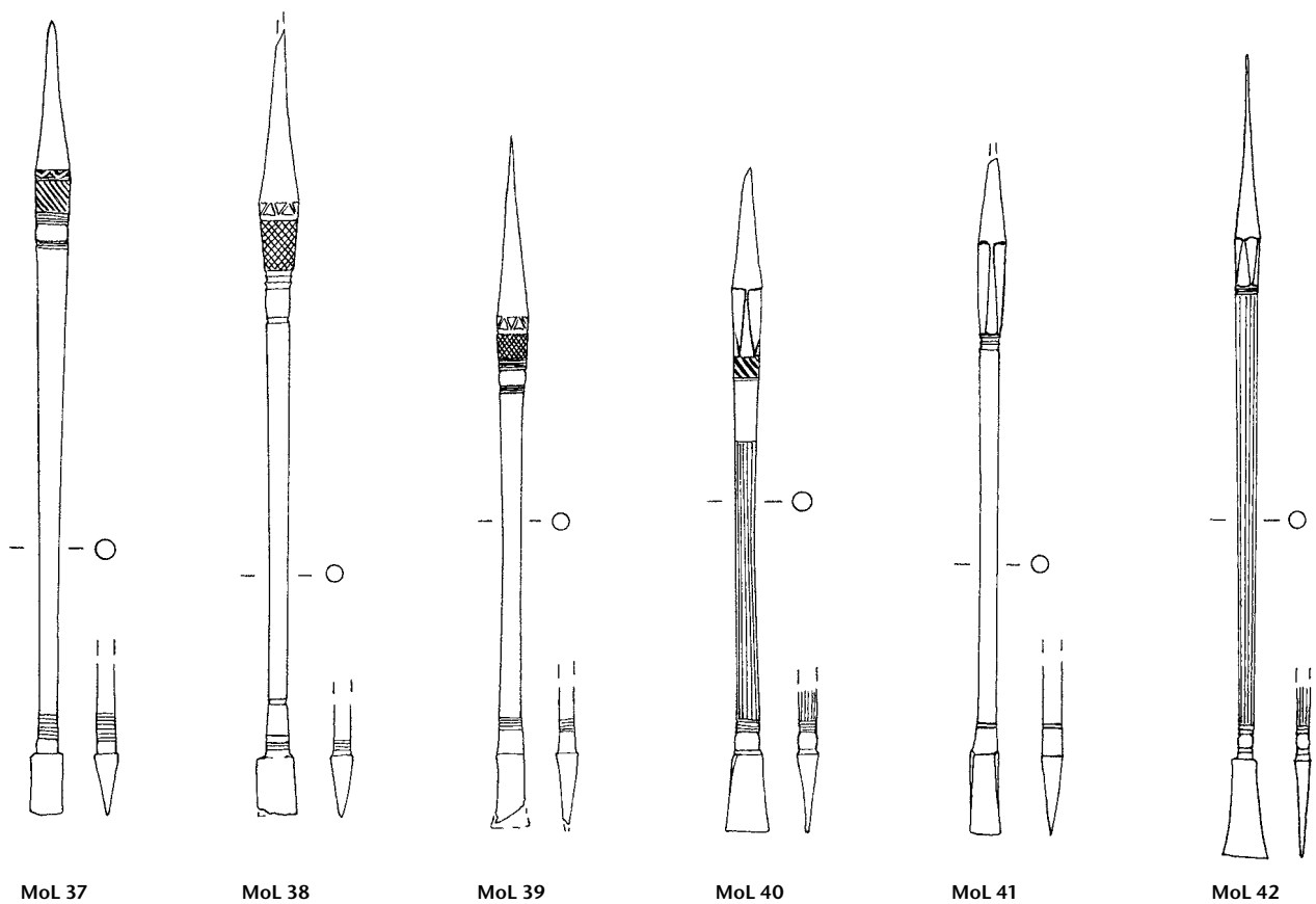
Tafel 188: Museum of London, London/GB. Formgruppe H 35: MoL 32–MoL 42. Eisen. M. 3:4.
