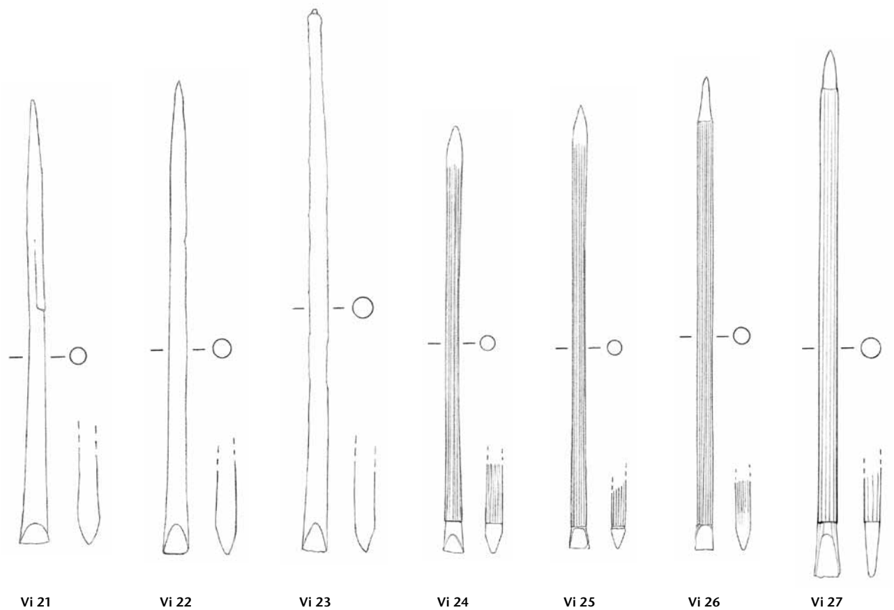
Tafel 120: Vindonissa. Formgruppe B 15 (Fortsetzung): Vi 13–Vi 18. Formgruppe B 16: Vi 21–Vi 27. Eisen. M. 3:4.
