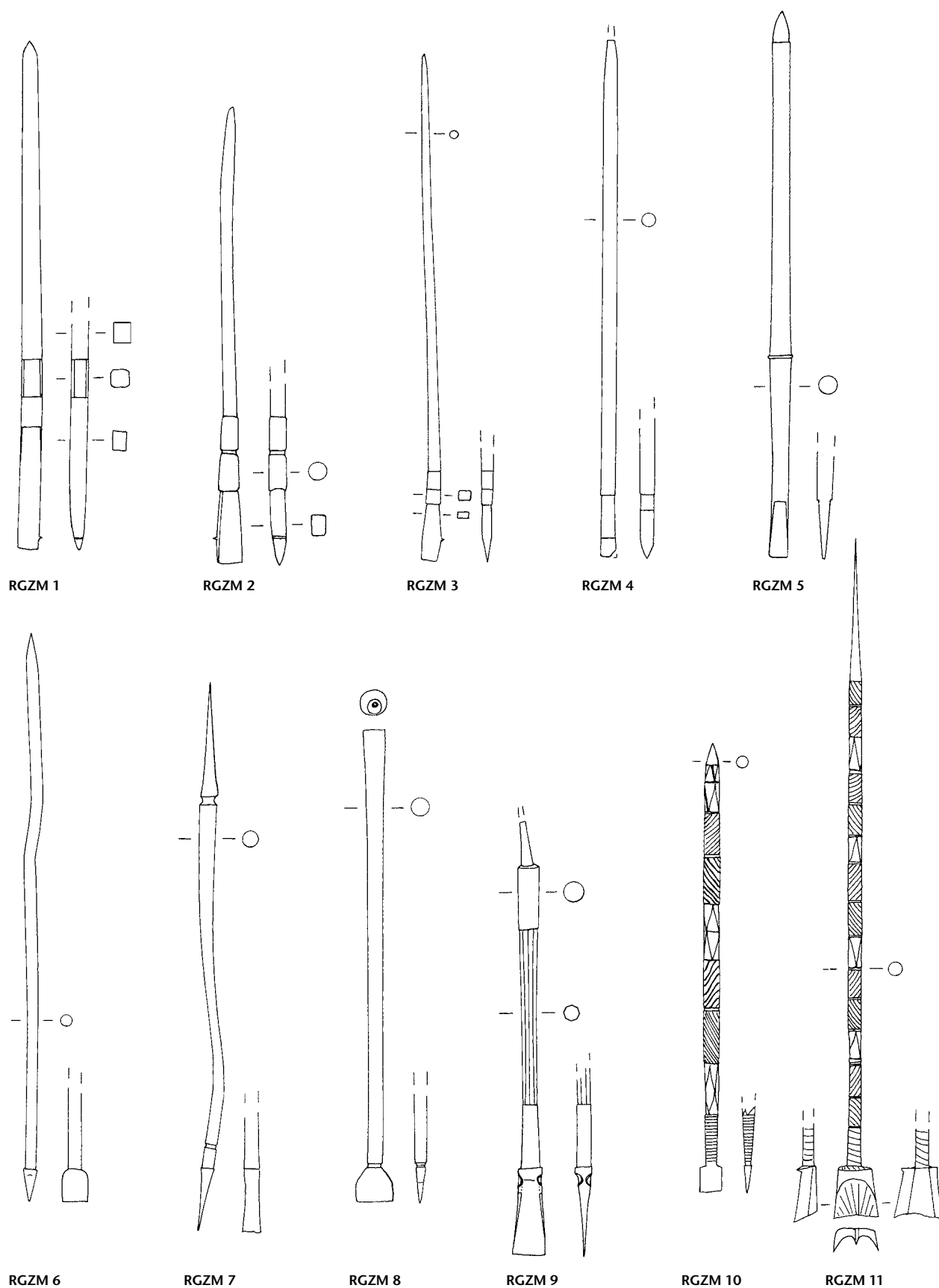
Tafel 177: Mainz/D und weitere Fundorte. Formgruppe B 15: RGZM 1–RGZM 5 . Formgruppe C 23: RGZM 6 . Formgruppe H 43: RGZM 7 . Formgruppe P 52: RGZM 8 . Formgruppe P 53: RGZM 9 . Formgruppe P 57: RGZM 10, RGZM 11 . Eisen ( RGZM 9, RGZM 10 Buntmetall). M. 3:4.
