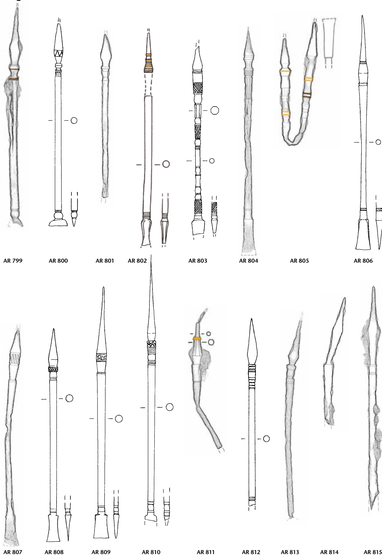
Tafel 53: Augusta Raurica. Formgruppe Q 68 (Fortsetzung): AR 799–AR 815. Eisen. M. 3:4.
