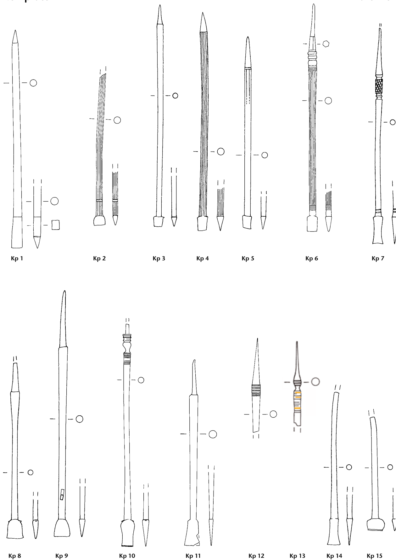
Tafel 164: Kempraten. Formgruppe B 15: Kp 1 . Formgruppe C 23: Kp 2 . Formgruppe C 24: Kp 3–Kp 5 . Formgruppe H 34: Kp 6 . Formgruppe H 43: Kp 7 . Formgruppe P 52: Kp 8, Kp 9 . Formgruppe P 55: Kp 10 . Formgruppe V 91: Kp 11 . Keiner Formgruppe zugewiesene Fragmente: Kp 12–Kp 15 . Eisen. M. 3:4.
