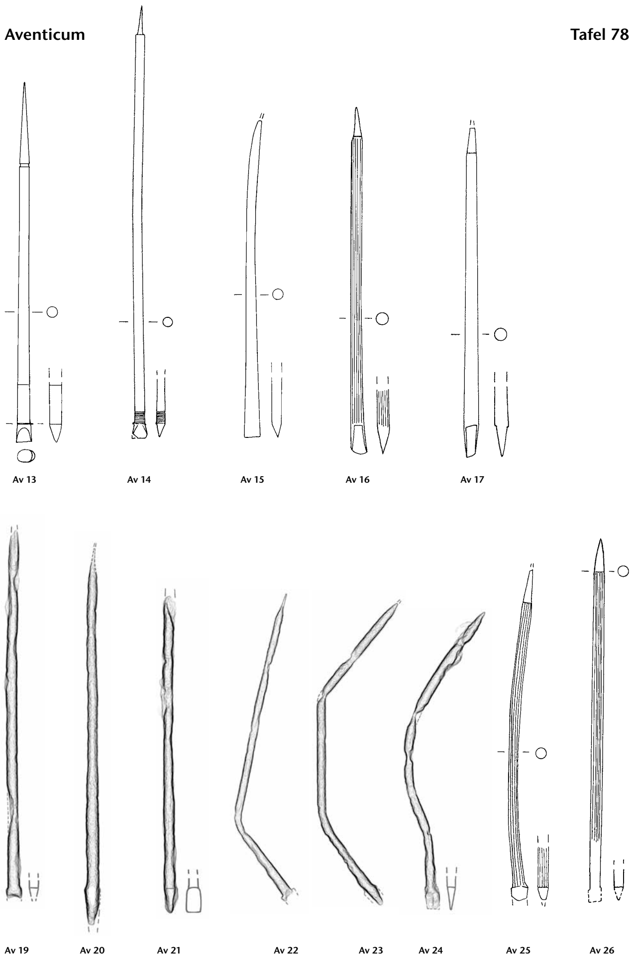
Tafel 78: Aventicum. Formgruppe B 16: Av 13–Av 17. Formgruppe C 22: Av 19–Av 26. Eisen. M. 3:4.
