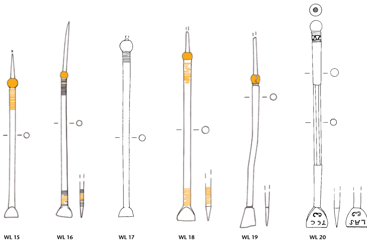
Tafel 180: Wiesbaden/D – Altfunde. Formgruppe P 55: WL 9, WL 10. Formgruppe P 56: WL 11. Formgruppe Q 68: WL 12. Formgruppe Q 69: WL 13, WL 14. Formgruppe Q 73: WL 15–WL 20. Eisen (WL 12, WL 20 Buntmetall). M. 3:4.
