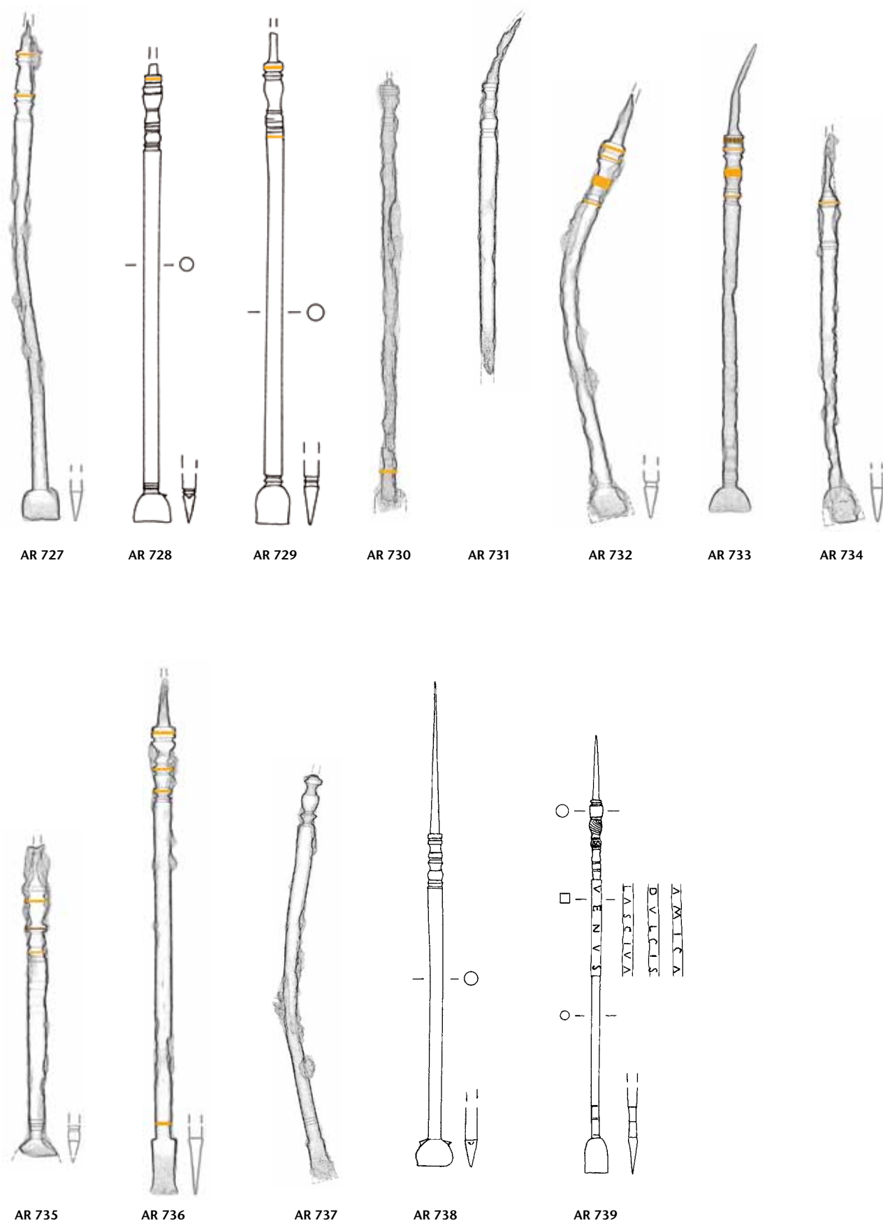
Tafel 48: Augusta Raurica. Formgruppe P 55: AR 727–AR 739. Eisen (AR 739 Buntmetall). M. 3:4.
