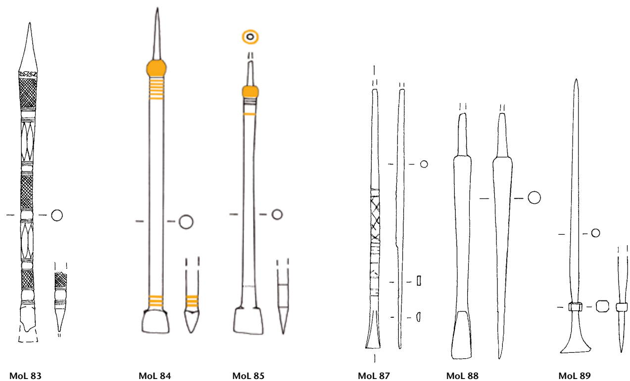
Tafel 192: Museum of London, London/GB. Formgruppe Q 68: MoL 76–MoL 79 . Formgruppe Q 70: MoL 80–MoL 82 . Formgruppe Q 71: MoL 83 . Formgruppe Q 73: MoL 84, MoL 85 . Keiner Formgruppe zuweisbare Stücke: MoL 87–MoL 89 . Eisen ( MoL 87 Buntmetall). M. 3:4.
