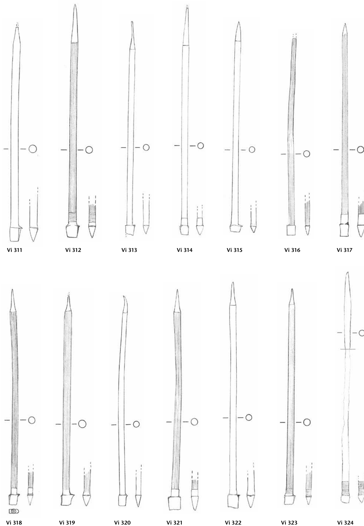
Tafel 142: Vindonissa. Formgruppe C 24 (Fortsetzung): Vi 311-Vi 324. Eisen. M. 3:4.
