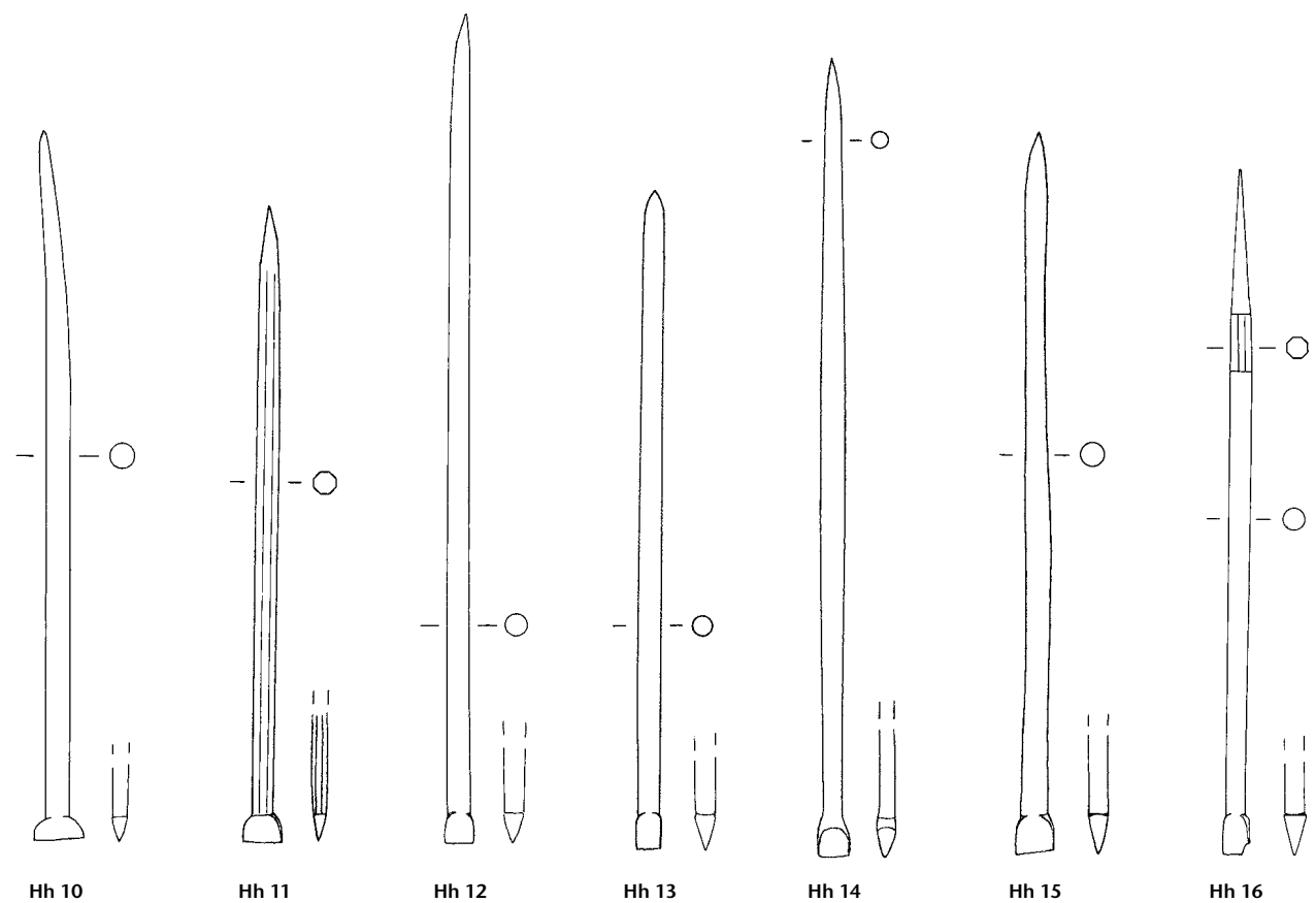
Tafel 173: Hofheim/D. Formgruppe B 15: Hh 1–Hh 7 . Formgruppe B 16: Hh 9 . Formgruppe C 23: Hh 10–Hh 16 . Eisen. M. 3:4.
