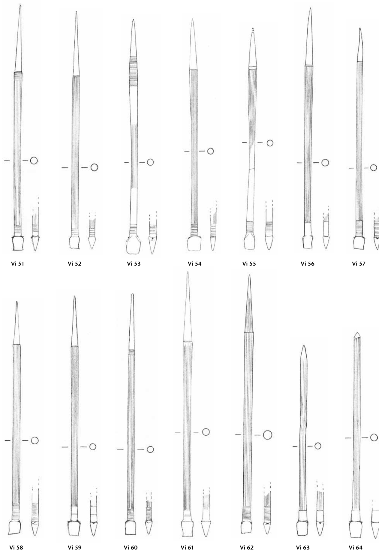
Tafel 123: Vindonissa. Formgruppe C 23 (Fortsetzung): Vi 51-Vi 64. Eisen. M. 3:4.
