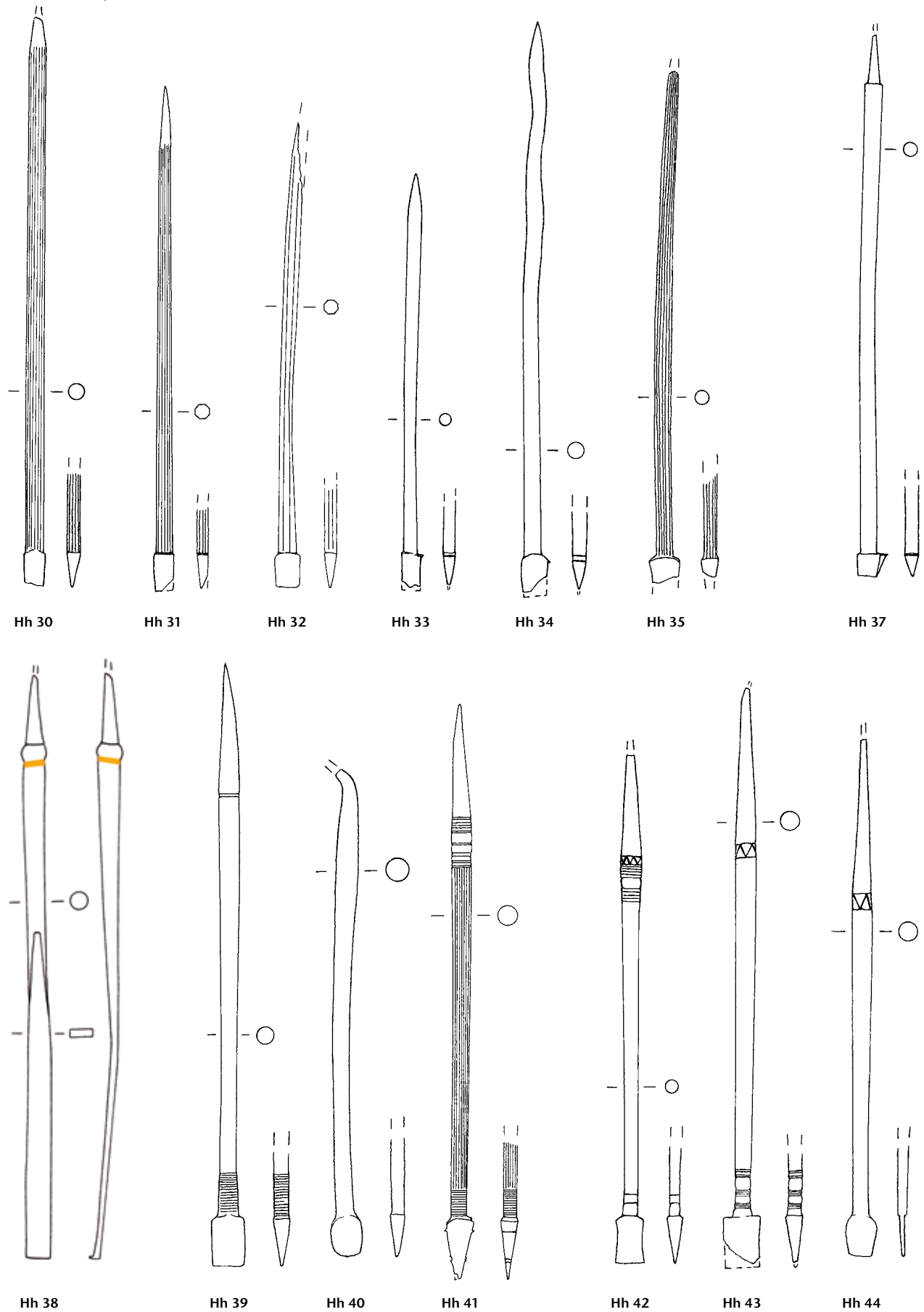
Tafel 175: Hofheim/D. Formgruppe C 24: Hh 30–Hh 35 . Formgruppe C 25: Hh 37 . Formgruppe H 32: Hh 38 . Formgruppe H 34: Hh 39–Hh 41 . Formgruppe H 35: Hh 42–Hh 44 . Eisen. M. 3:4.
