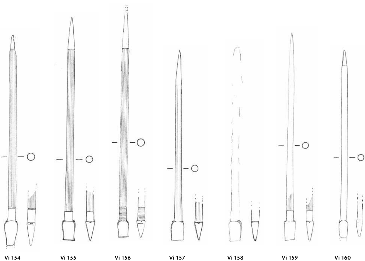
Tafel 130: Vindonissa. Formgruppe C 23 (Fortsetzung): Vi 148–Vi 160. Eisen. M. 3:4.
