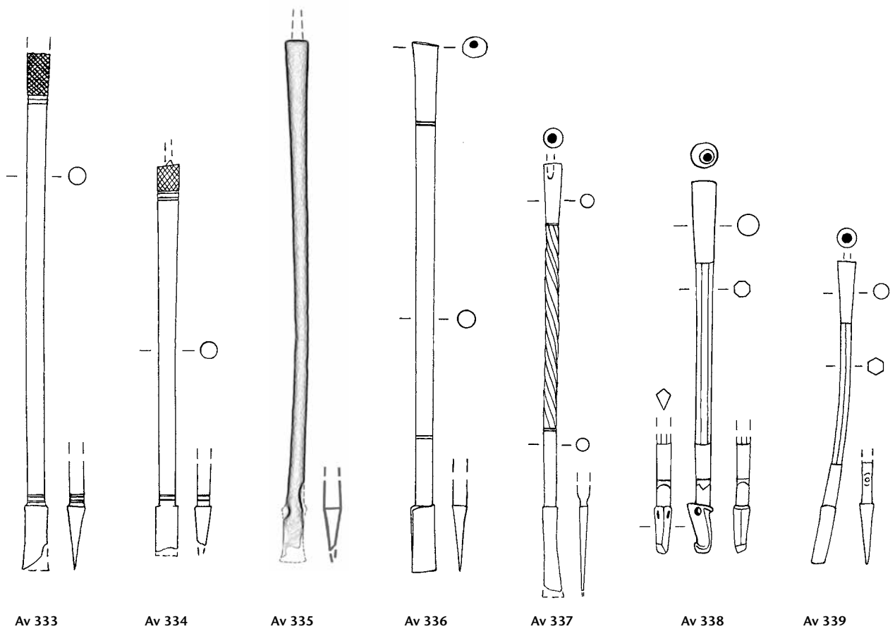
Tafel 102: Aventicum. Formgruppe P 51: Av 325–Av 332. Formgruppe P 52: Av 333–Av 339. Eisen (Av 337–Av 339 Buntmetall). M. 3:4.
