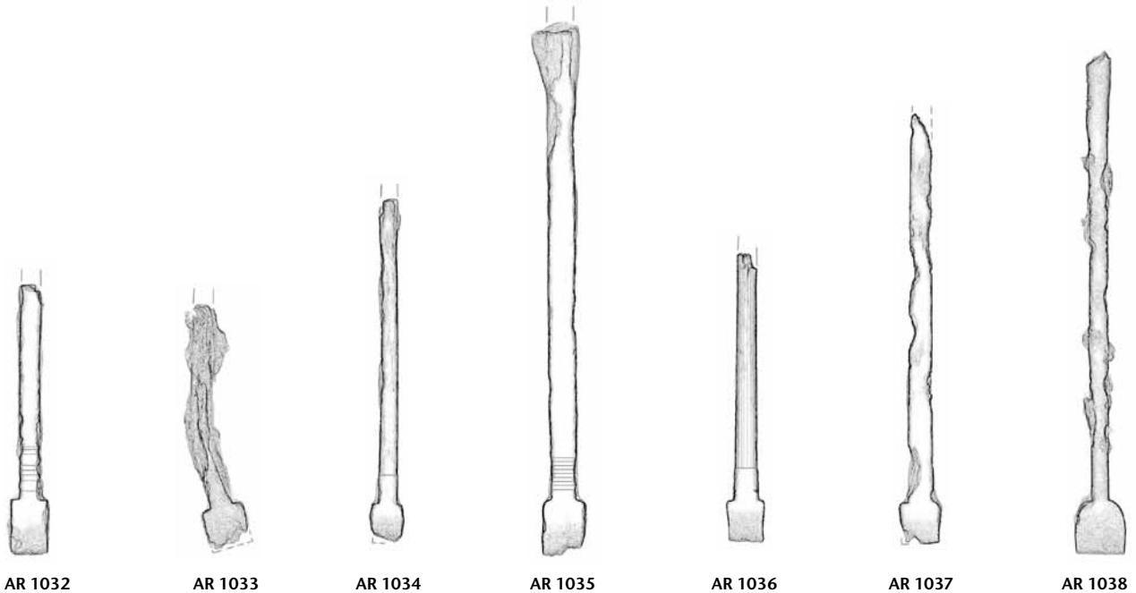
Tafel 67: Augusta Raurica. Nicht mehr zuweisbare fragmentierte Schreibgriffel sowie Spitzen- und Spatelfragmente, 1.–2. Jh. n. Chr. (Fortsetzung): AR 1032–AR 1038. Eisen. M. 3:4.
