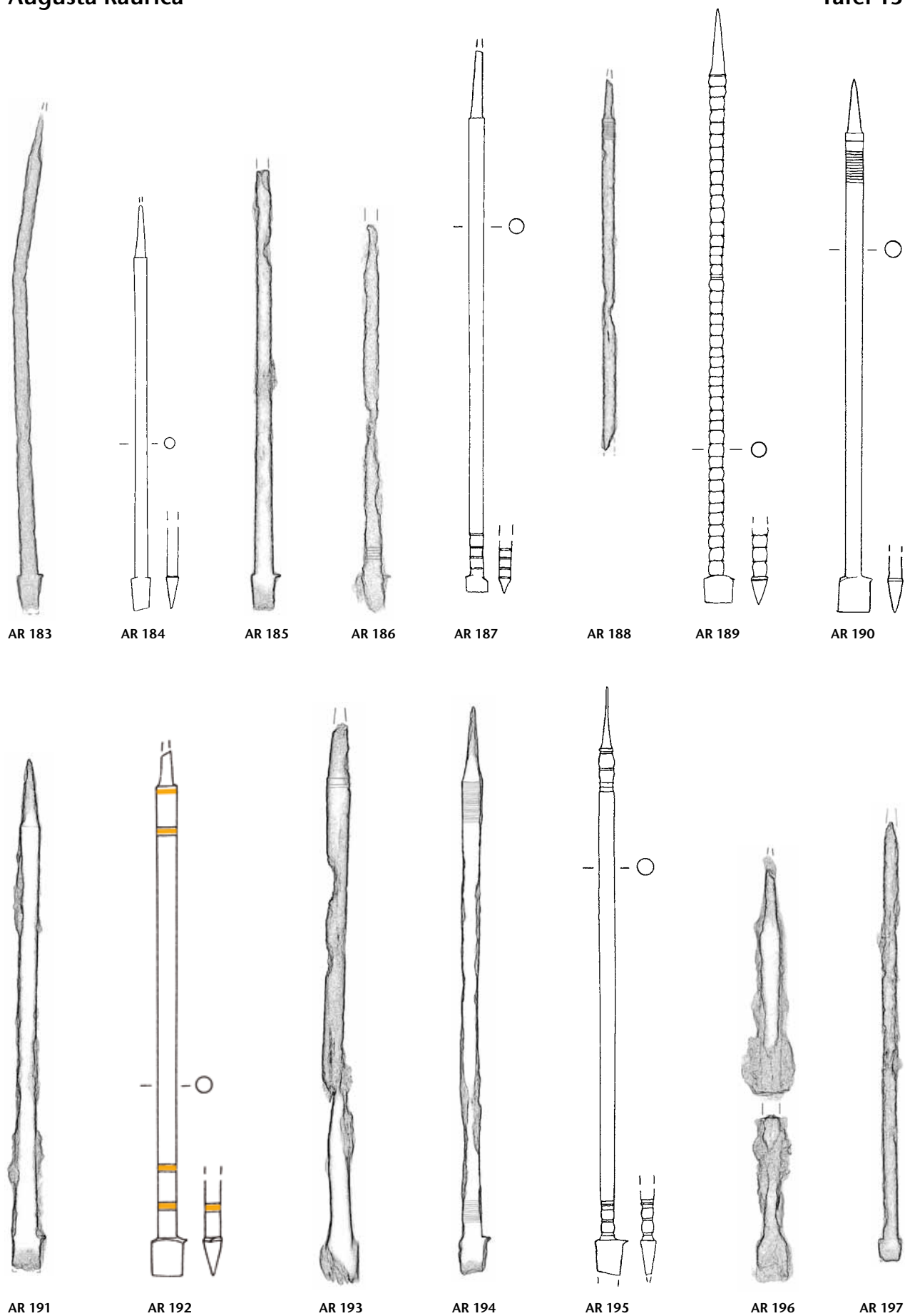
Tafel 13: Augusta Raurica. Formgruppe C 24 (Fortsetzung): AR 183–AR 197. Eisen. M. 3:4.
