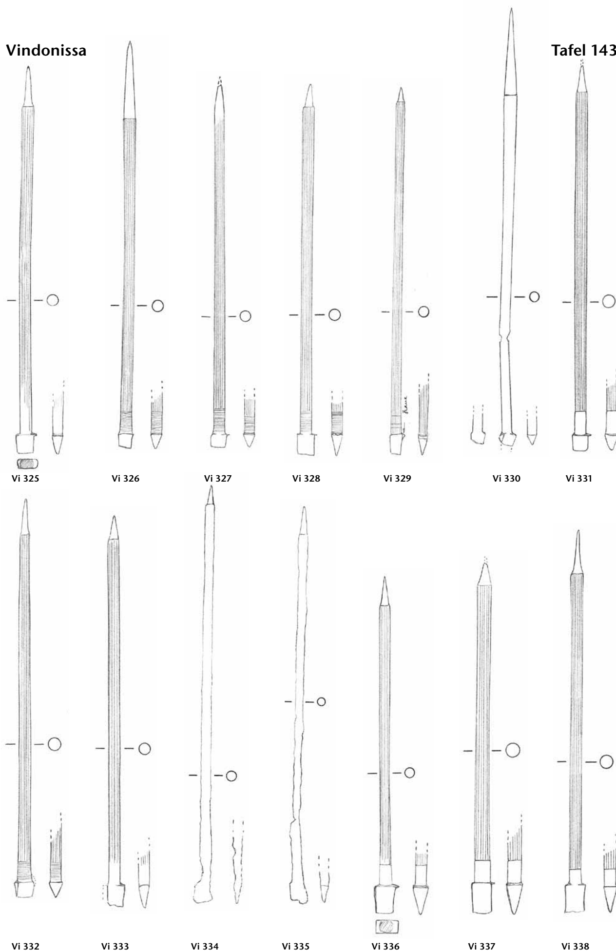
Tafel 143: Vindonissa. Formgruppe C 24 (Fortsetzung): Vi 325-Vi 338. Eisen. M. 3:4.
