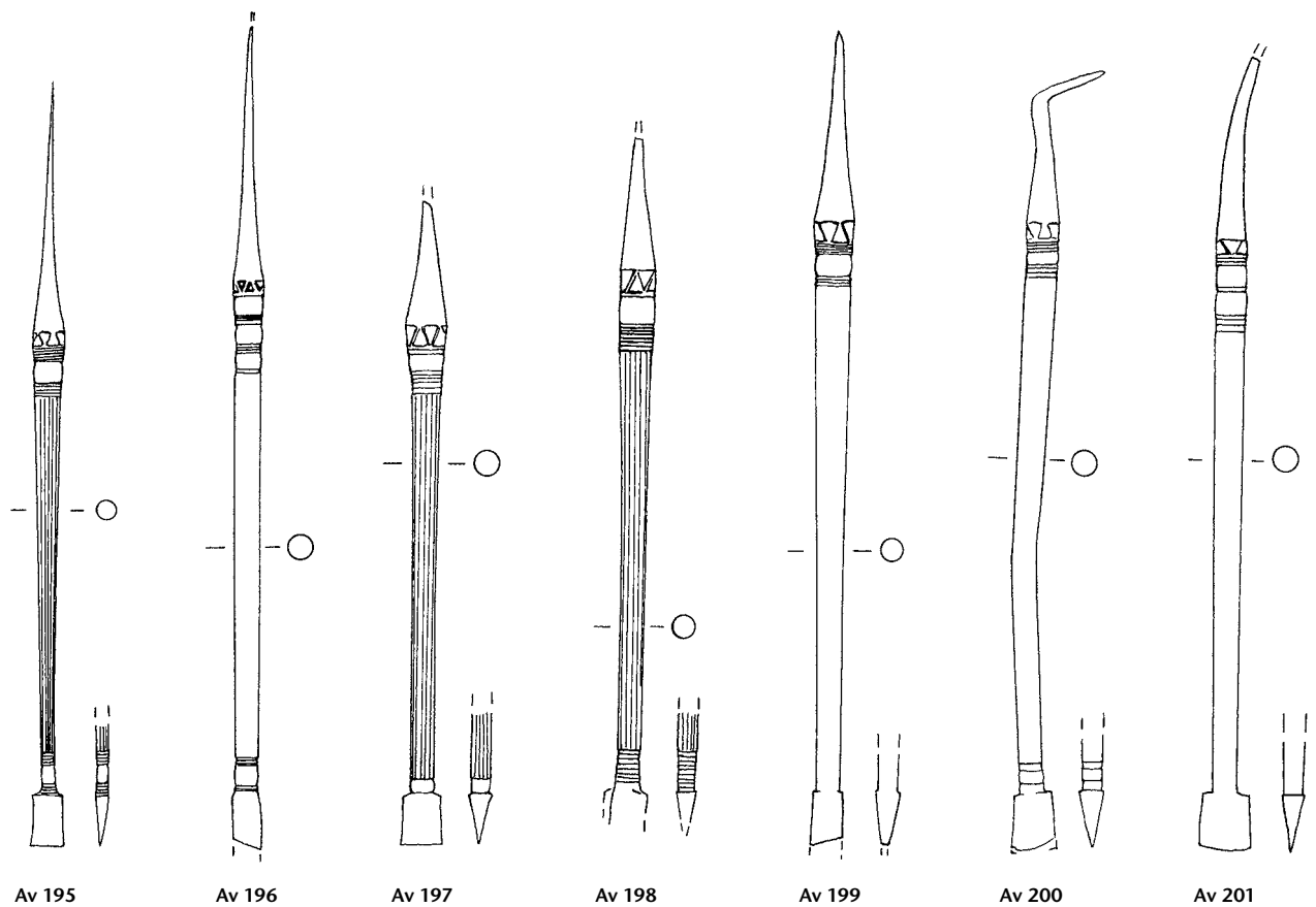
Tafel 91: Aventicum. Formgruppe H 35: Av 189–Av 201. Eisen. M. 3:4.
