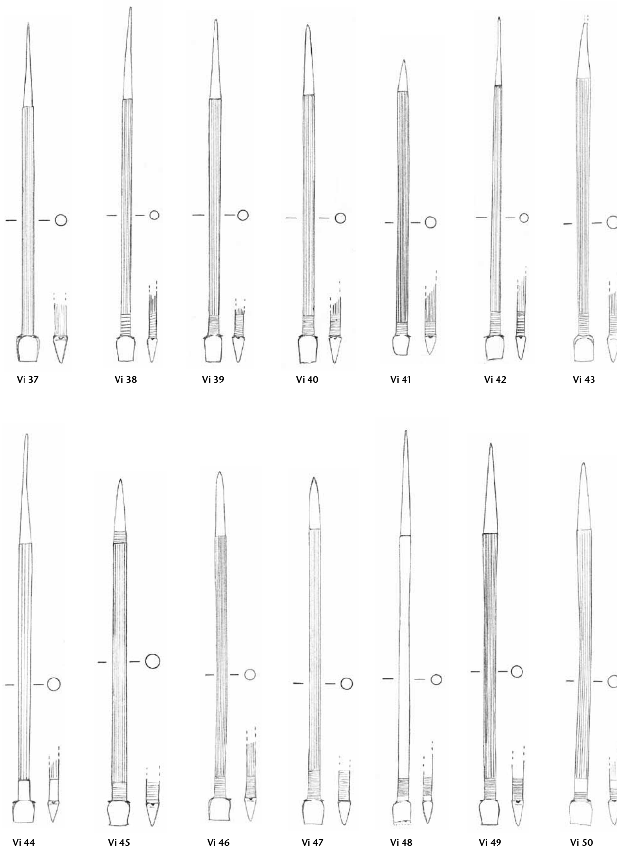
Tafel 122: Vindonissa. Formgruppe C 23: Vi 37-Vi 50. Eisen. M. 3:4.
