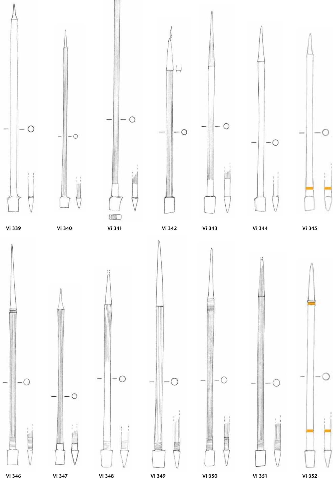
Tafel 144: Vindonissa. Formgruppe C 24 (Fortsetzung): Vi 339–Vi 352. Eisen. M. 3:4.
