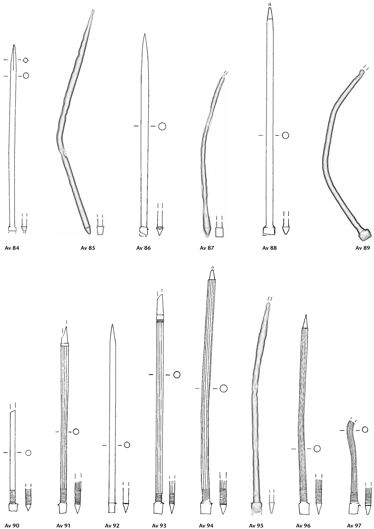
Tafel 83: Aventicum. Formgruppe C 24: Av 84–Av 97. Eisen. M. 3:4.
