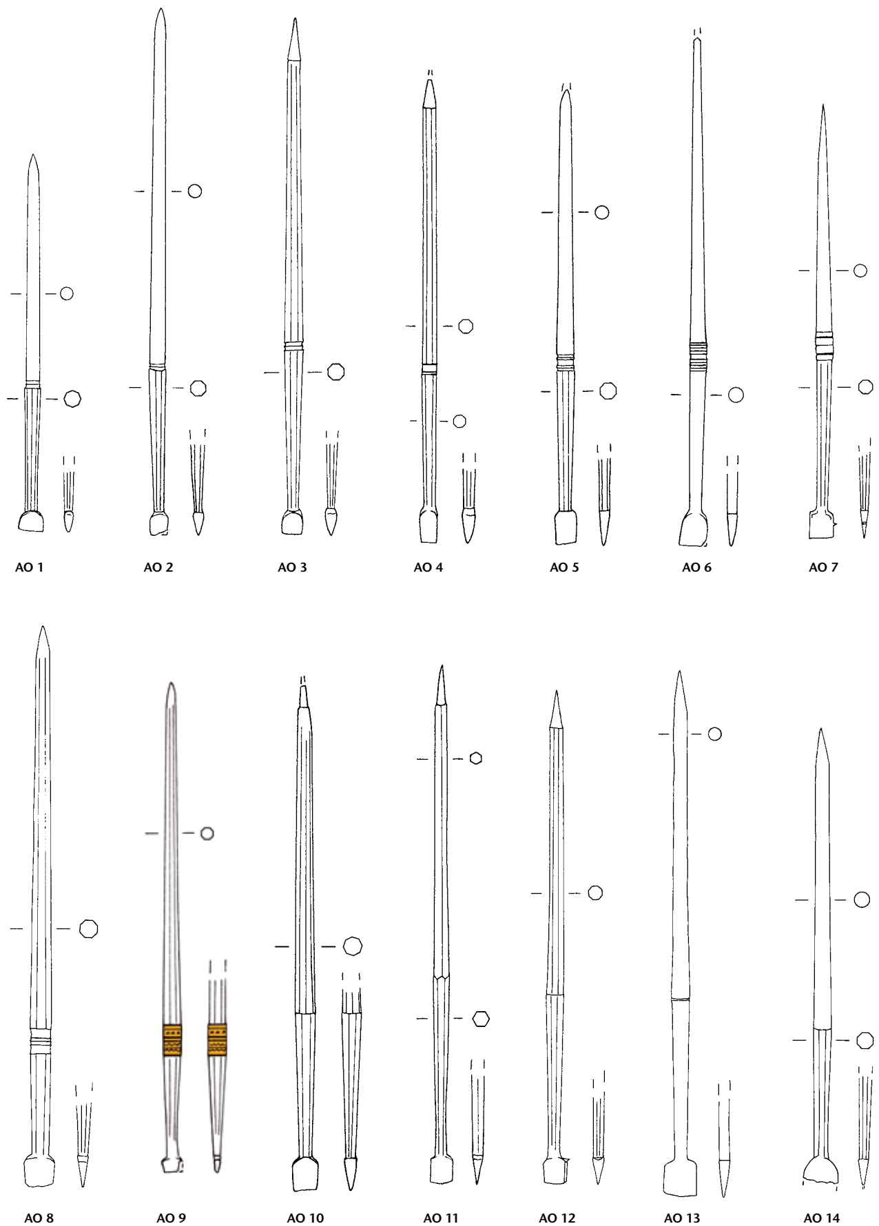
Tafel 168: Augsburg-Oberhausen/D. Formgruppe A 10: AO 1-AO 14. Eisen. M. 3:4.
