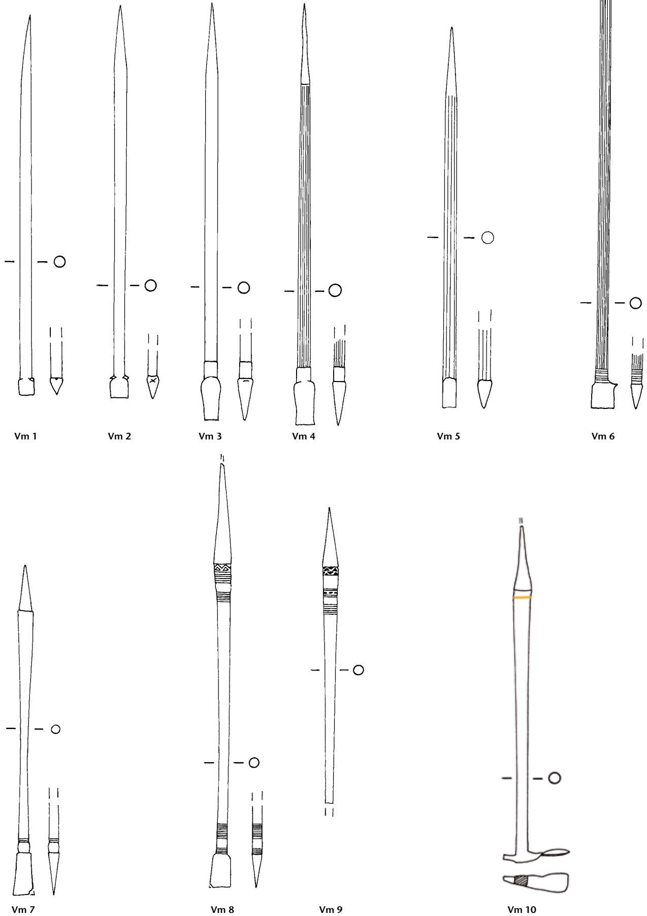
Tafel 183: Verulamium – St Albans/GB. Formgruppe C 23: Vm 1-Vm 4. Formgruppe C 24: Vm 5. Formgruppe C 25: Vm 6. Formgruppe H 34: Vm 7. Formgruppe H 35: Vm 8, Vm 9. Formgruppe H 40: Vm 10. Eisen. M. 3:4.
