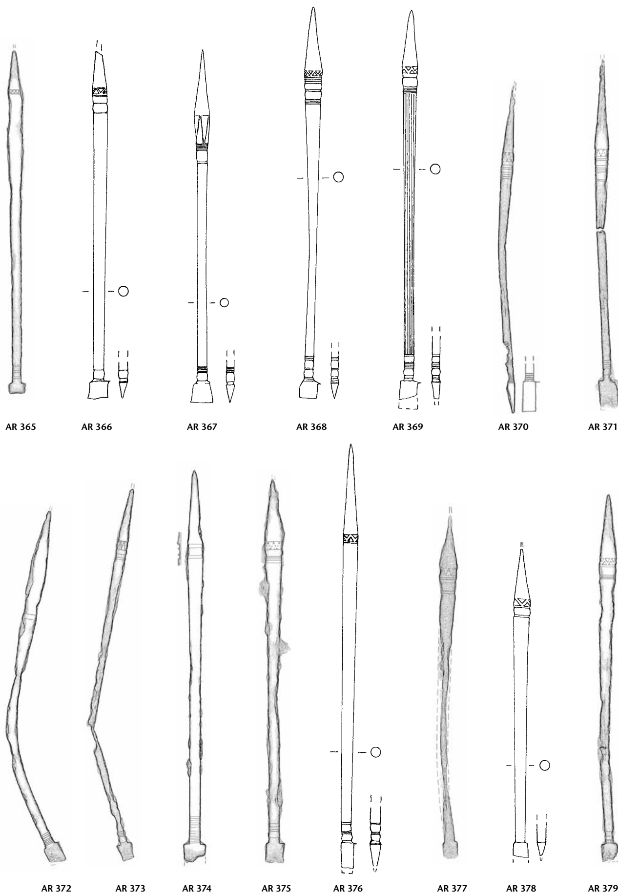
Tafel 24: Augusta Raurica. Formgruppe H 35: AR 365–AR 379. Eisen. M. 3:4.
