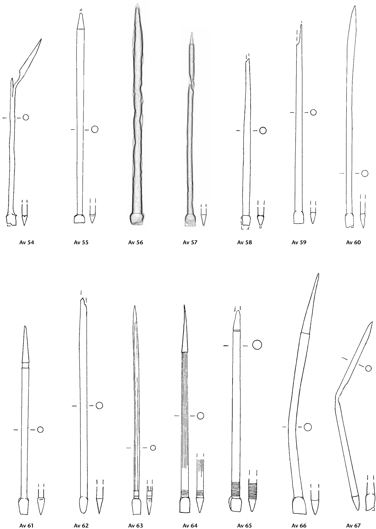
Tafel 81: Aventicum. Formgruppe C 23 (Fortsetzung): Av 54–Av 67. Eisen. M. 3:4.
