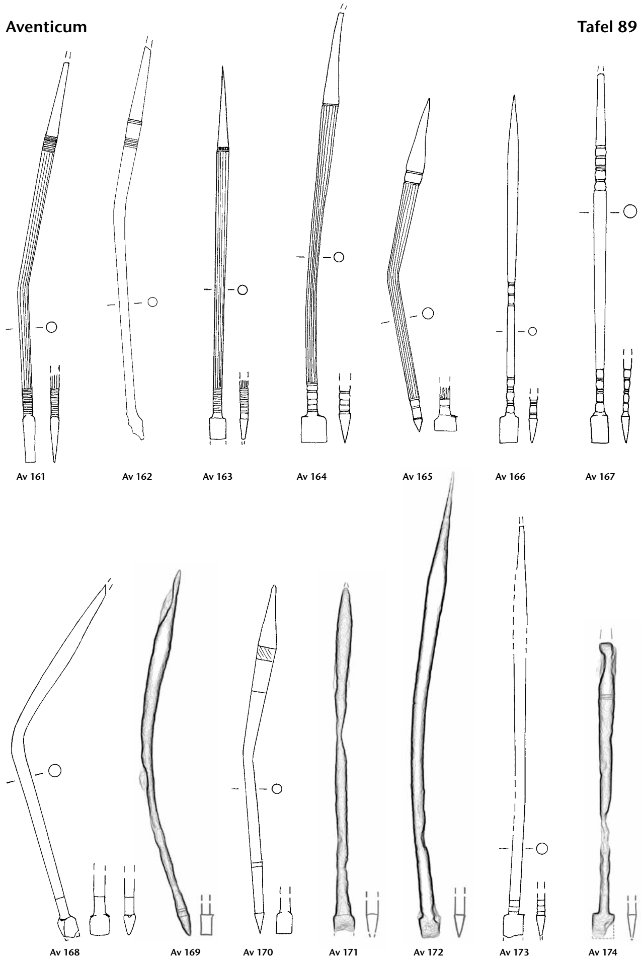
Tafel 89: Aventicum. Formgruppe H 34 (Fortsetzung): Av 161–Av 174. Eisen. M. 3:4.
