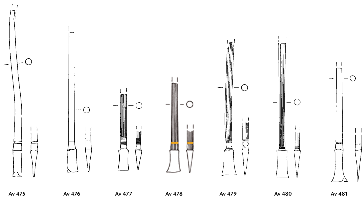
Tafel 113: Aventicum. Nicht mehr zuweisbare Spatel- und Schaftfragmente: Av 465–Av 481. Eisen (Av 477 Buntmetall). M. 3:4.
