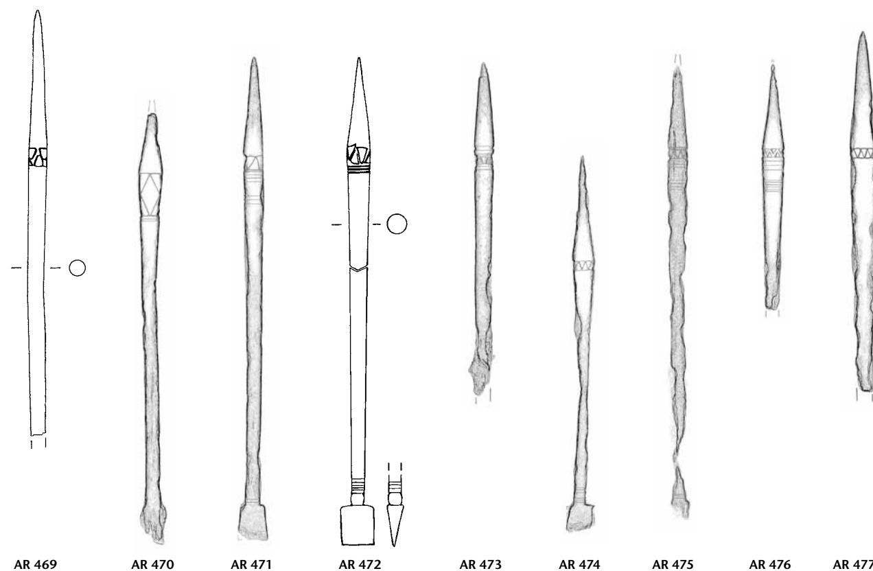
Tafel 30: Augusta Raurica. Formgruppe H 35 (Fortsetzung): AR 461–AR 477. Eisen. M. 3:4.
