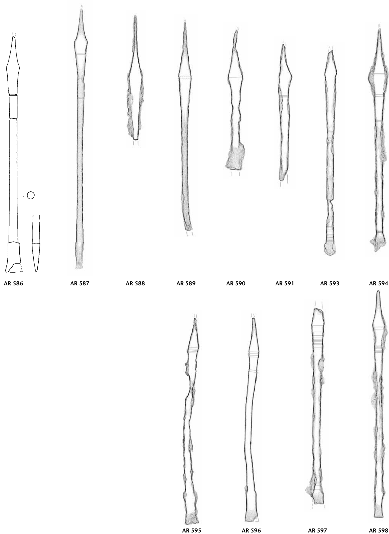
Tafel 38: Augusta Raurica. Formgruppe H 47 (Fortsetzung): AR 586–AR 594. Formgruppe P 51: AR 595–AR 598. Eisen. M. 3:4.
