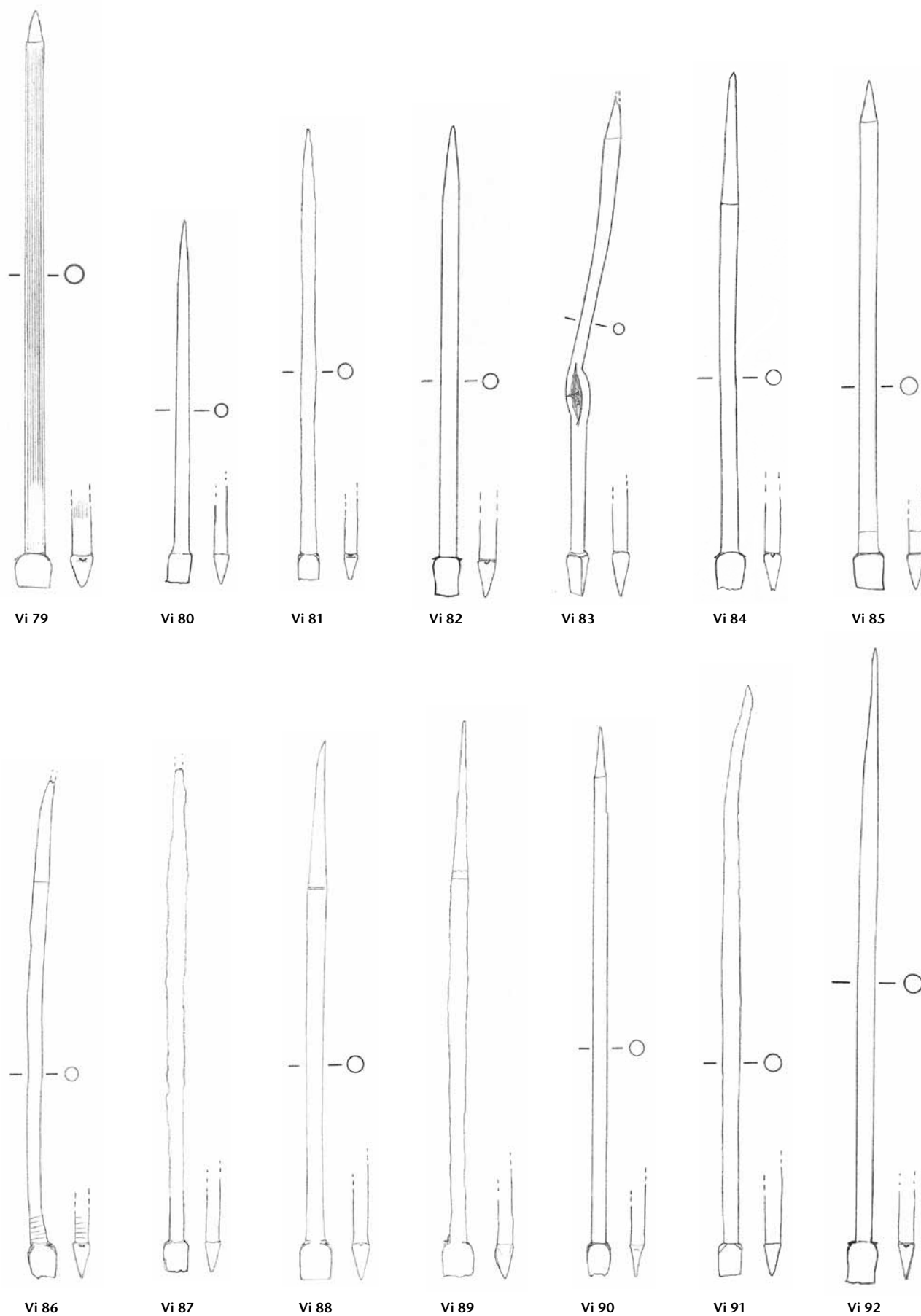
Tafel 125: Vindonissa. Formgruppe C 23 (Fortsetzung): Vi 79–Vi 92. Eisen. M. 3:4.
