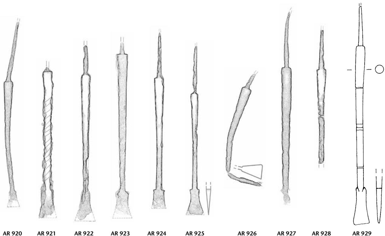
Tafel 62: Augusta Raurica. Formgruppe V 91: AR 920–AR 929. Eisen (AR 929 Buntmetall). M. 3:4.
