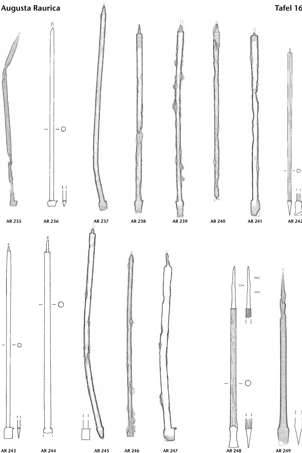
Tafel 16: Augusta Raurica. Formgruppe C 25: AR 235–AR 247. Formgruppe C 26: AR 248, AR 249. Eisen. M. 3:4.
