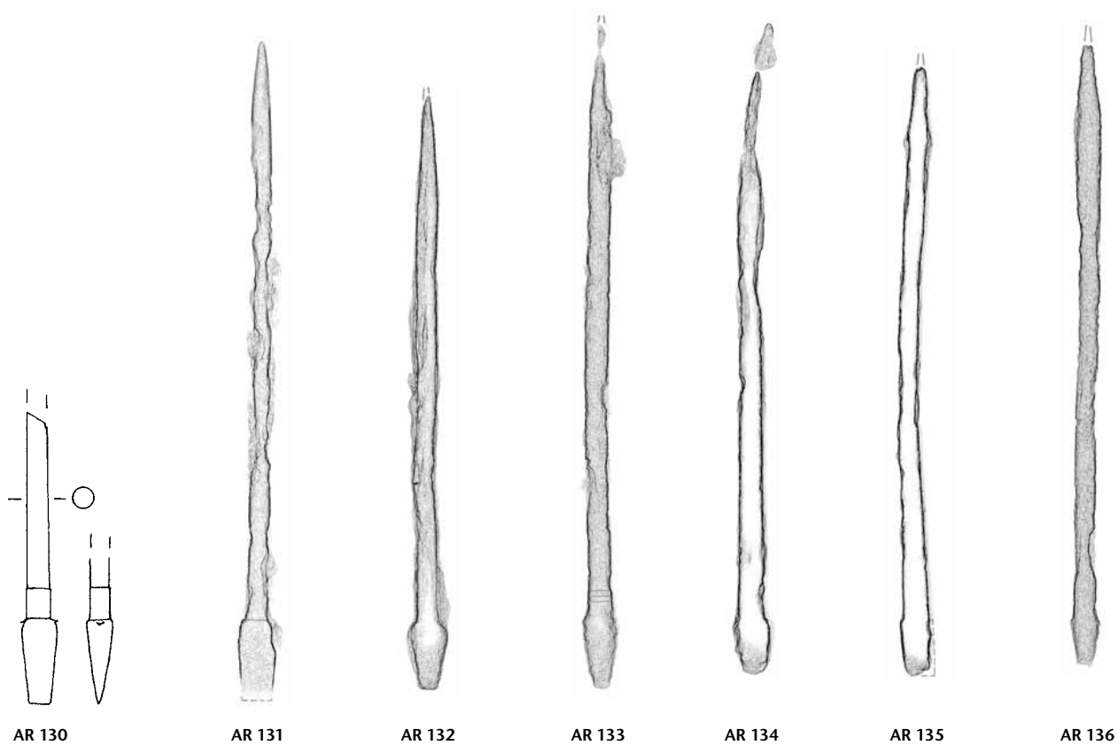
Tafel 9: Augusta Raurica, Formgruppe C 23 (Fortsetzung): AR 122–AR 136. Eisen. M. 3:4.
