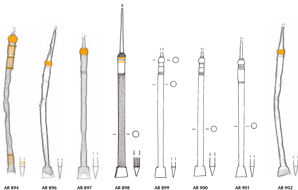
Tafel 60: Augusta Raurica. Formgruppe Q 73: AR 886–AR 902. Eisen. M. 3:4.
