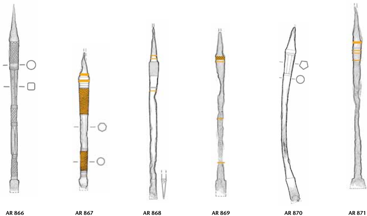
Tafel 58: Augusta Raurica. Formgruppe Q 71 (Fortsetzung): AR 866–AR 871. Eisen. M. 3:4.
