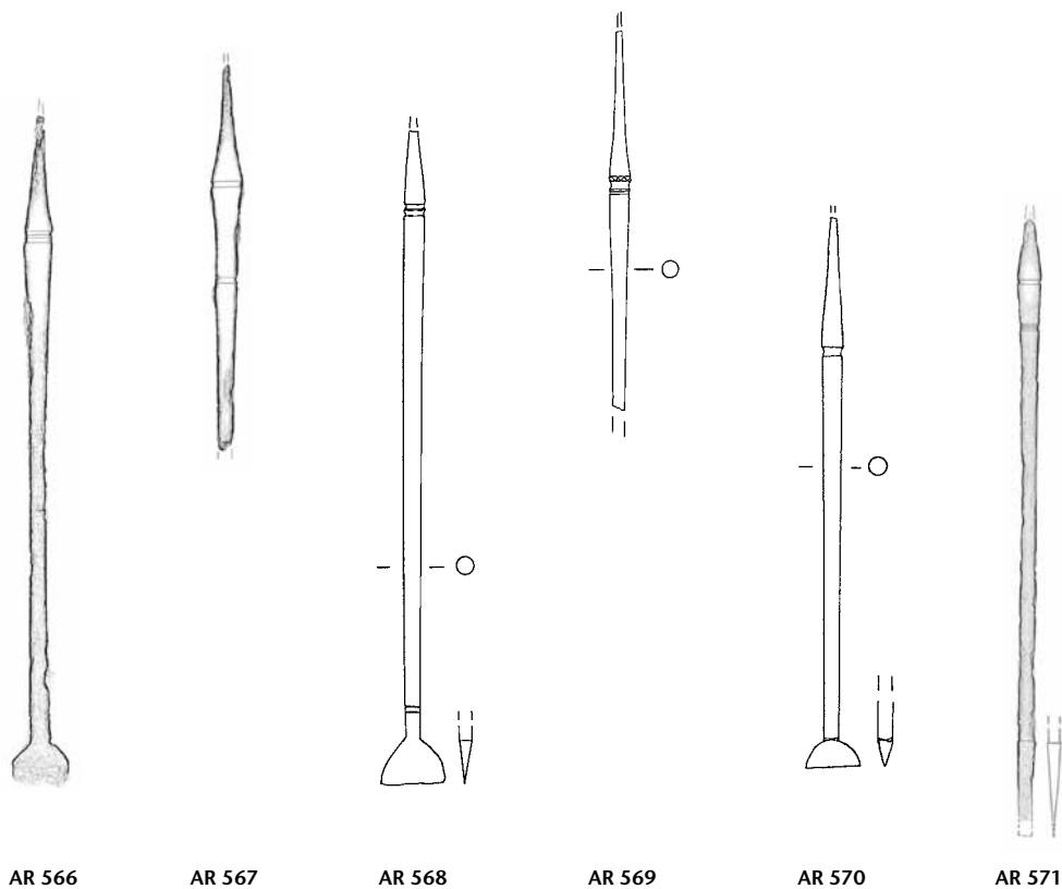
Tafel 36: Augusta Raurica. Formgruppe H 43 (Fortsetzung): AR 566–AR 571. Eisen. M. 3:4.
