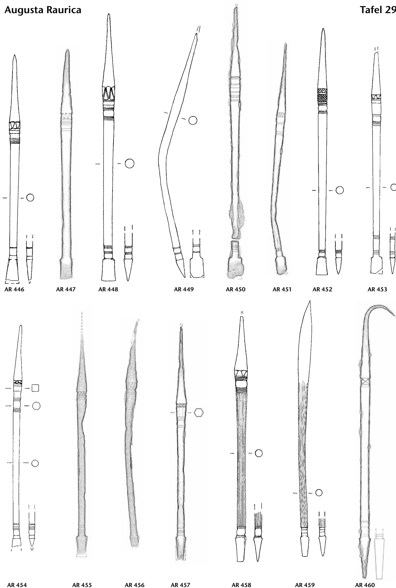
Tafel 29: Augusta Raurica. Formgruppe H 35 (Fortsetzung): AR 446–AR 460. Eisen. M. 3:4.
