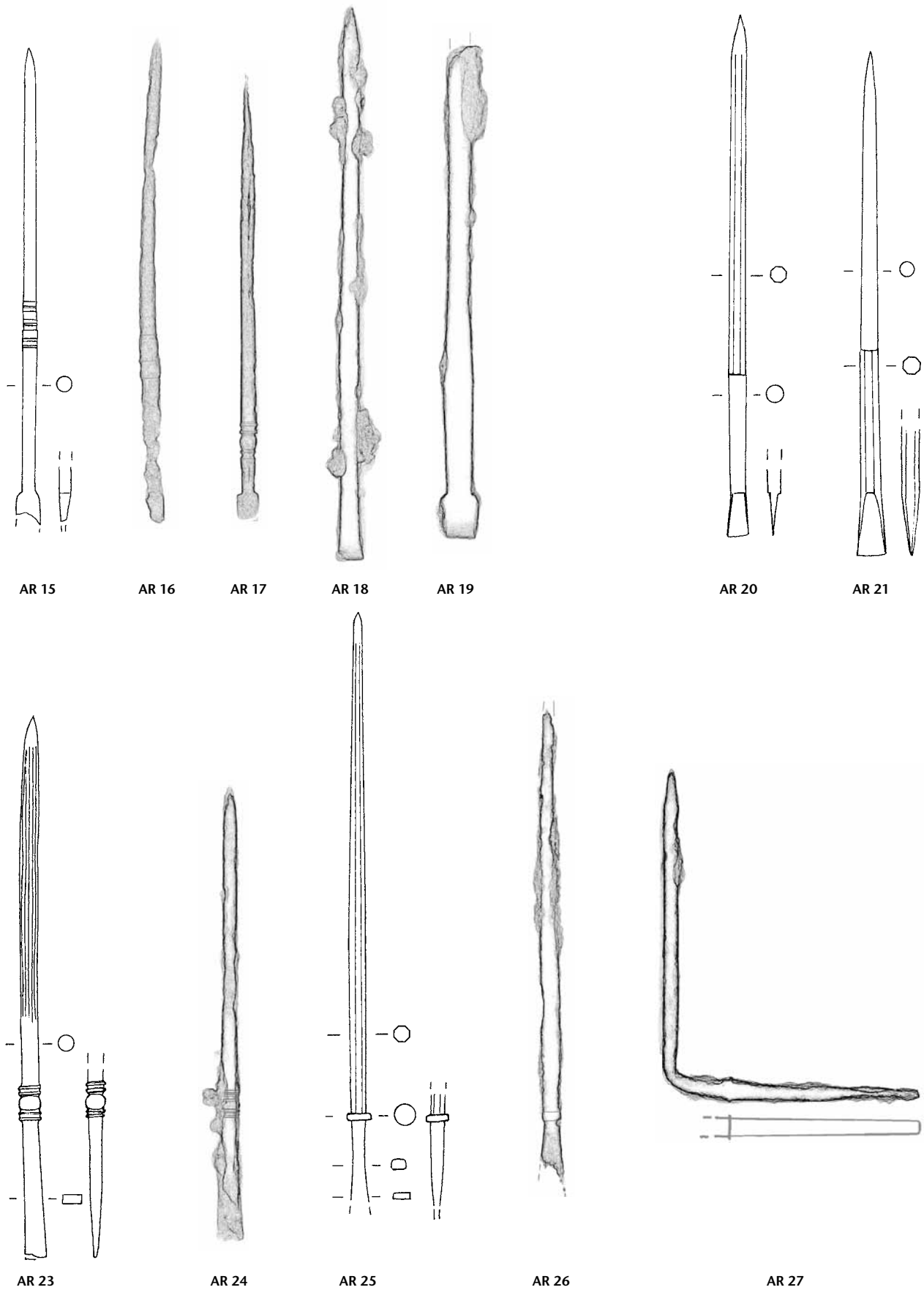
Tafel 2: Augusta Raurica. Formgruppe A 10 (Fortsetzung): AR 15–AR 19. Formgruppe A 11: AR 20, AR 21. Formgruppe A 12: AR 23–AR 27. Eisen. M. 3:4.
