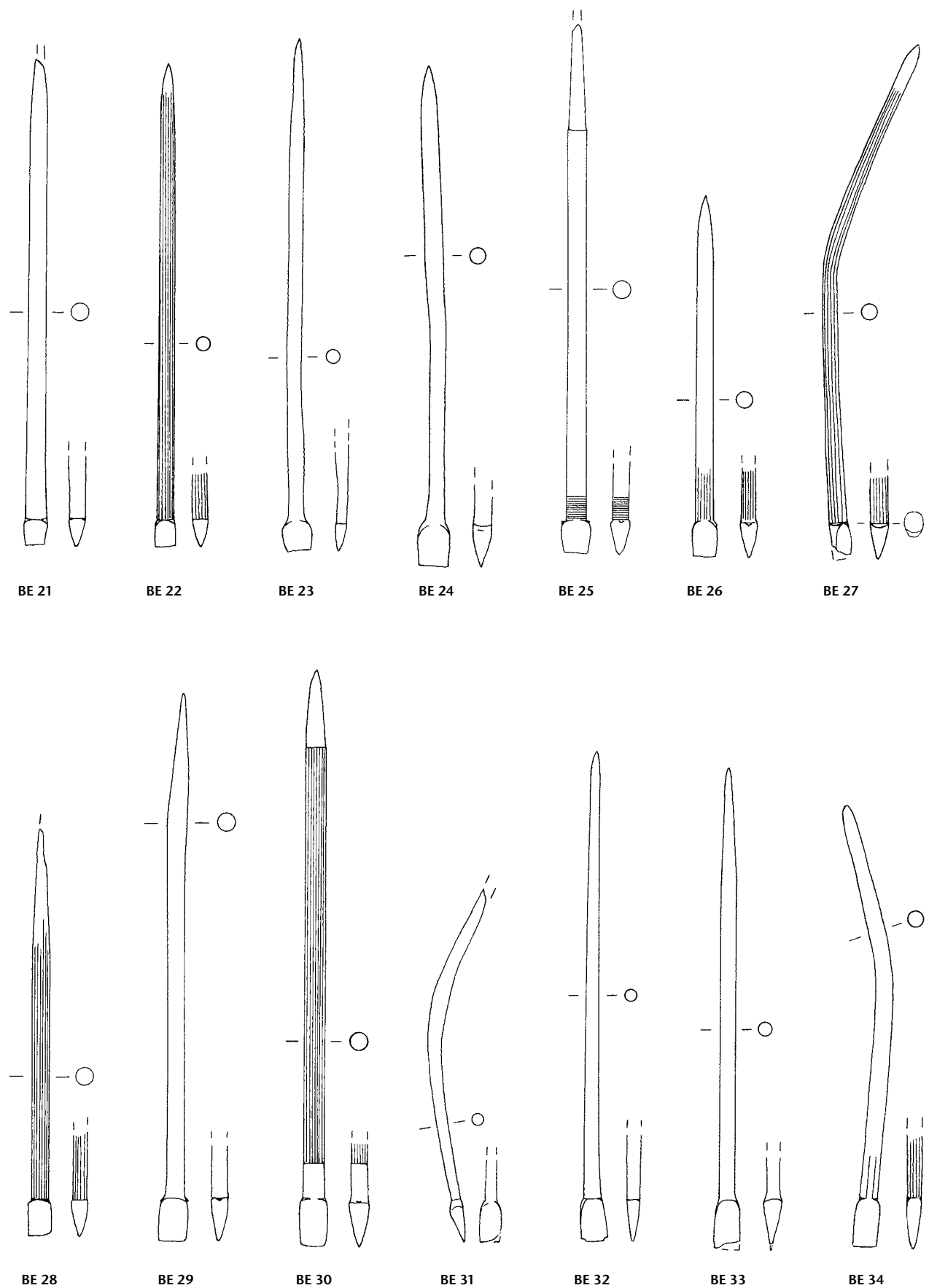
Tafel 157: Bern-Engelhalbinsel. Formgruppe C 23: BE 21–BE 34. Eisen. M. 3:4.
