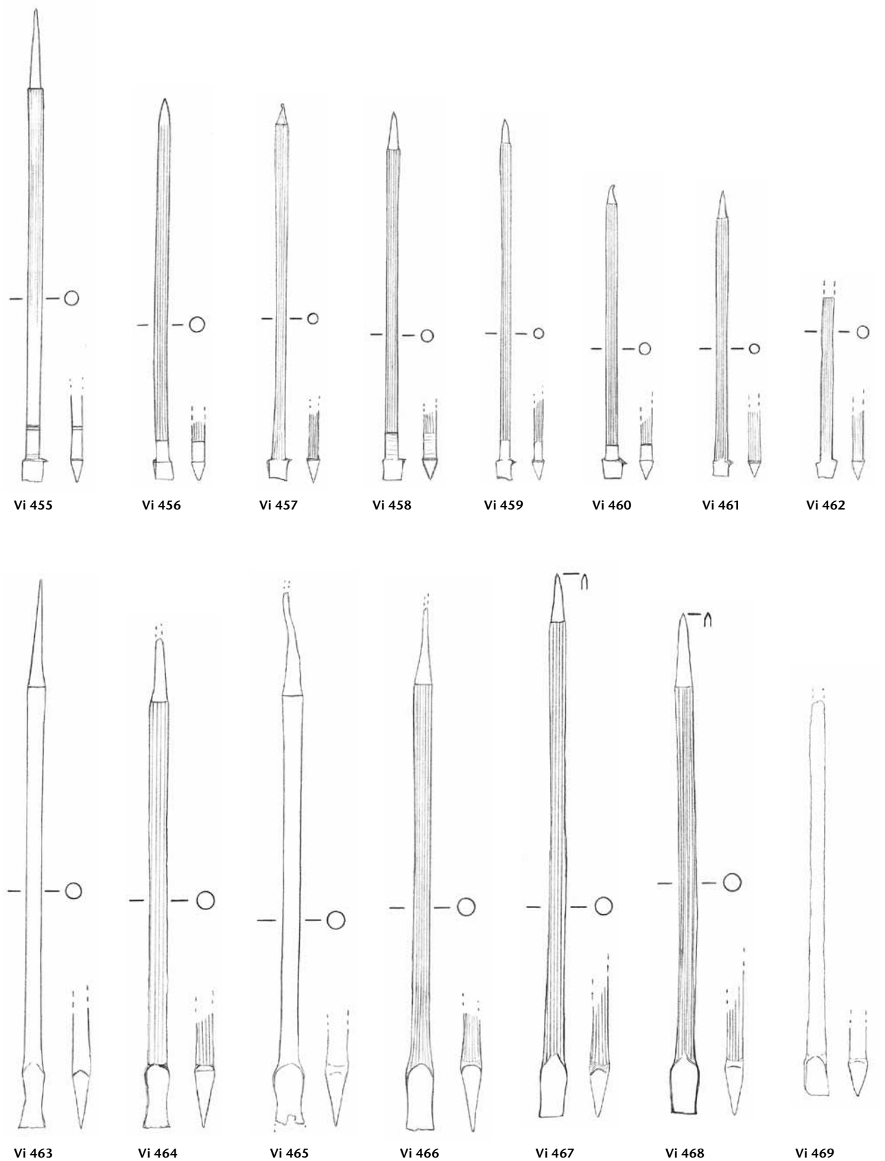
Tafel 153: Vindonissa. Formgruppe C 25 (Fortsetzung): Vi 455–Vi 462. Formgruppe C 26: Vi 463–Vi 469. Eisen. M. 3:4.
