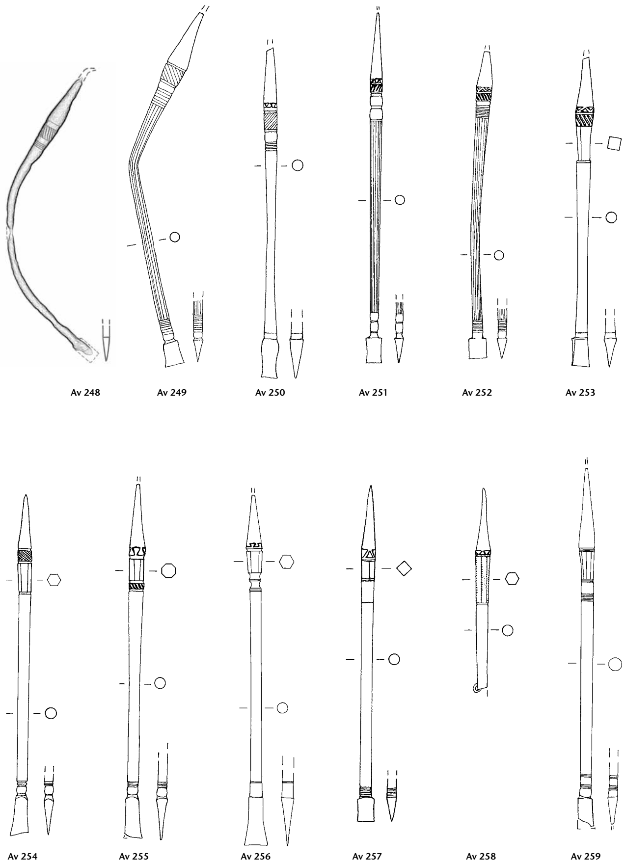
Tafel 96: Aventicum. Formgruppe H 35 (Fortsetzung): Av 248–Av 259. Eisen. M. 3:4.
