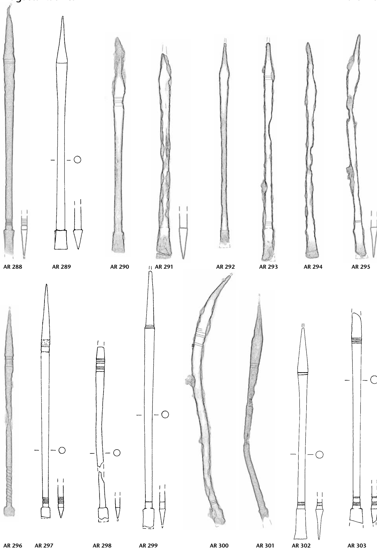
Tafel 20: Augusta Raurica. Formgruppe H 34 (Fortsetzung): AR 288–AR 303. Eisen. M. 3:4.
