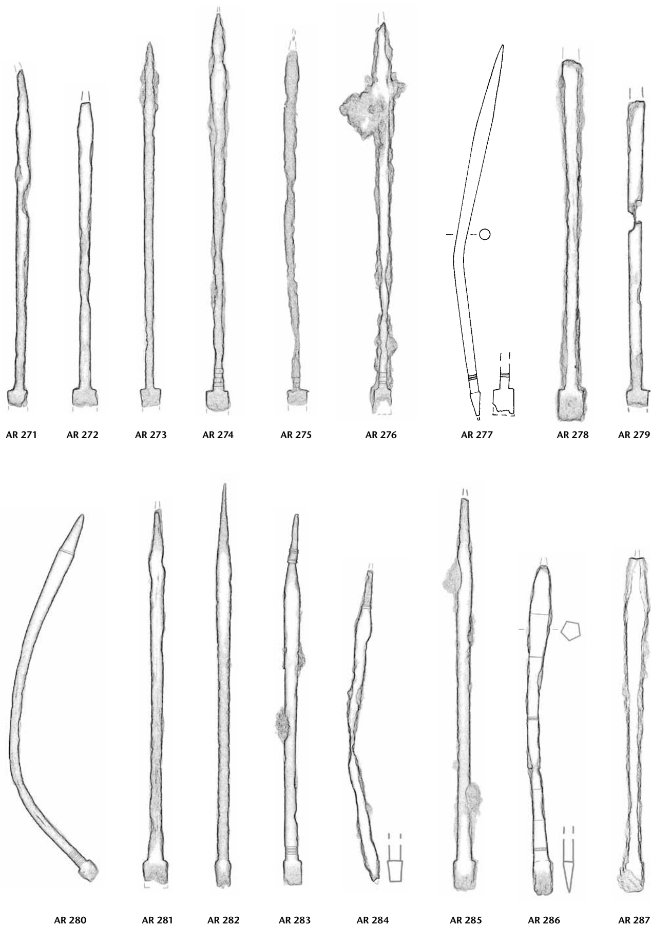
Tafel 19: Augusta Raurica. Formgruppe H 34: AR 271–AR 287. Eisen. M. 3:4.
