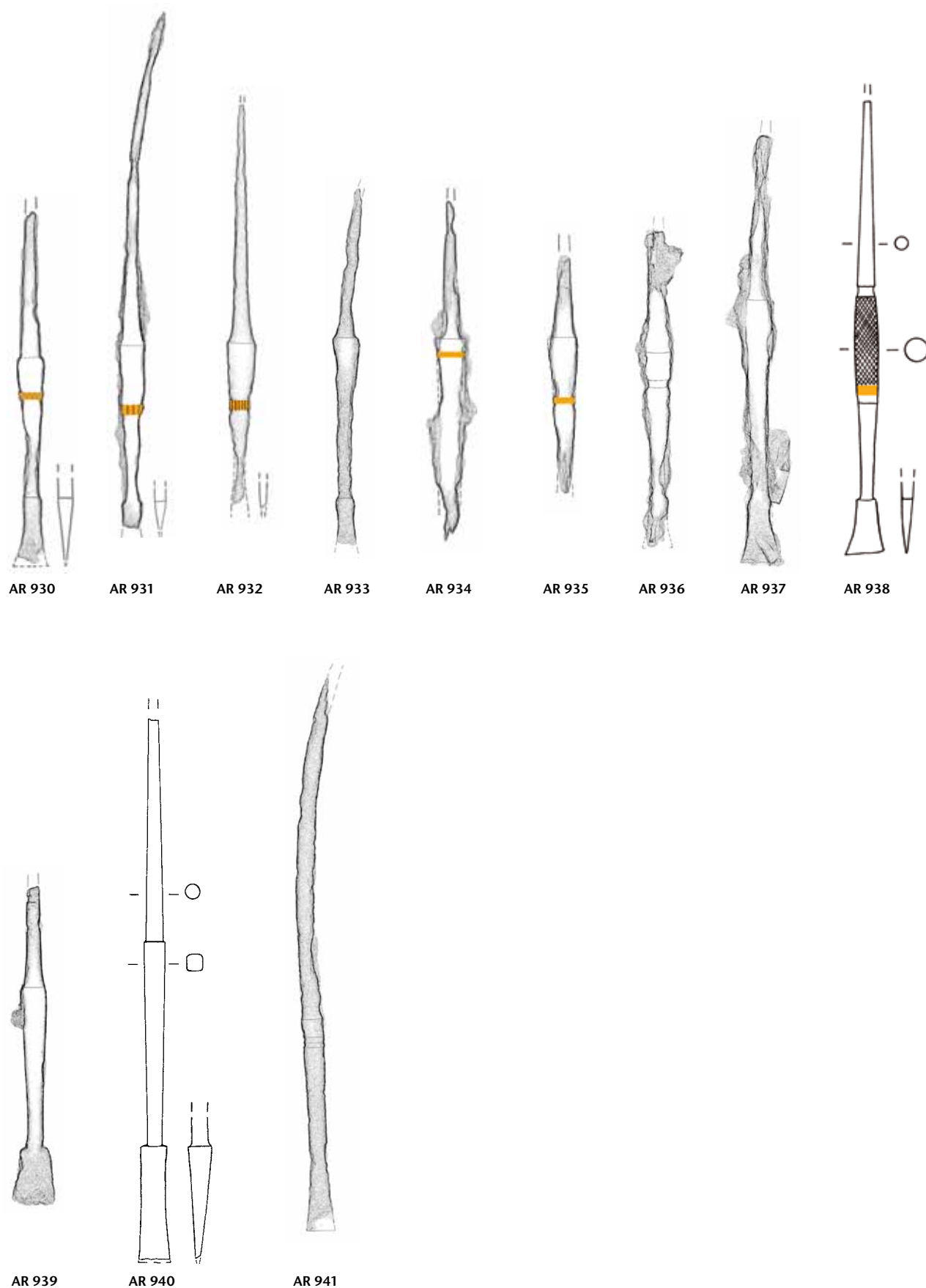
Tafel 63: Augusta Raurica. Formgruppe V 92: AR 930–AR 941. Eisen. M. 3:4.
