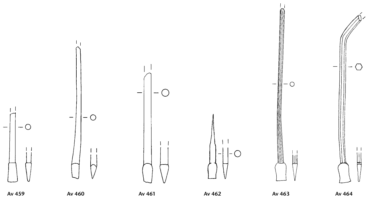
Tafel 112: Aventicum. Nicht mehr zuweisbare Spatel- und Schaftfragmente: Av 452–Av 464. Eisen (Av 459 Buntmetall). M. 3:4.
