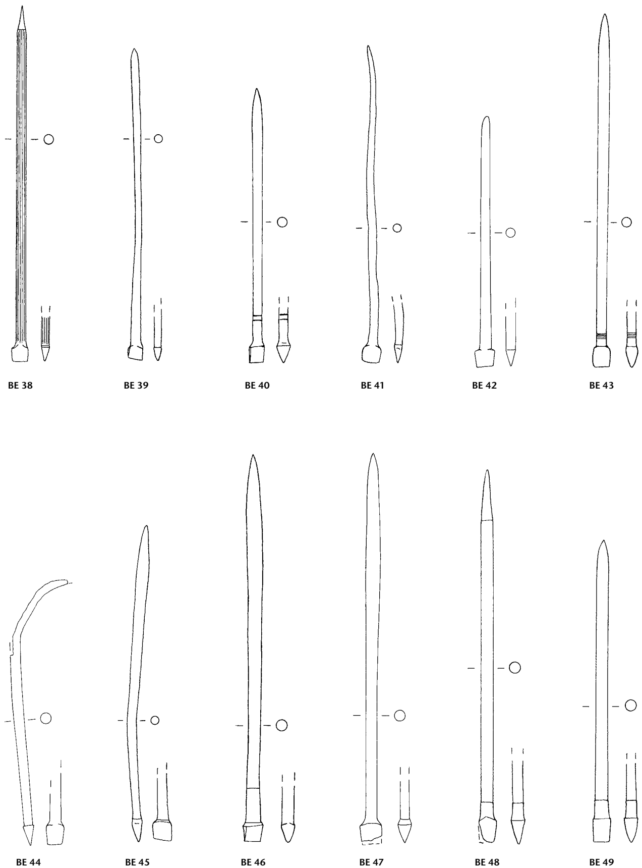
Tafel 158: Bern-Engelhalbinsel. Formgruppe C 24: BE 38–BE 49. Eisen. M. 3:4.
