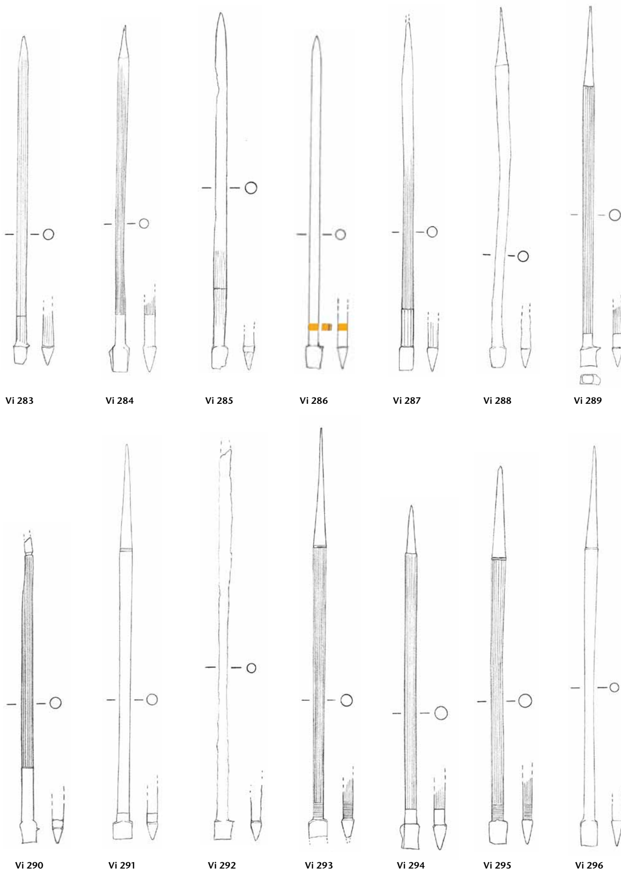
Tafel 140: Vindonissa. Formgruppe C 24 (Fortsetzung): Vi 283–Vi 296. Eisen. M. 3:4.
