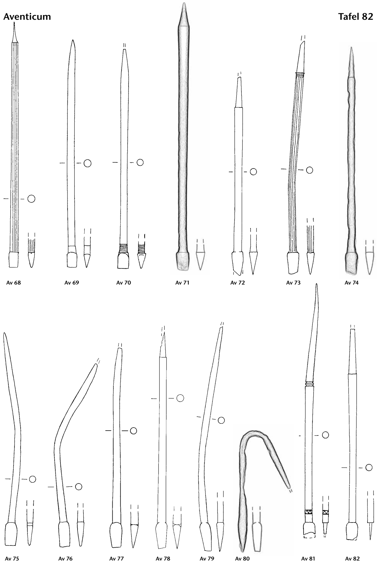
Tafel 82: Aventicum. Formgruppe C 23 (Fortsetzung): Av 68–Av 82. Eisen. M. 3:4.
