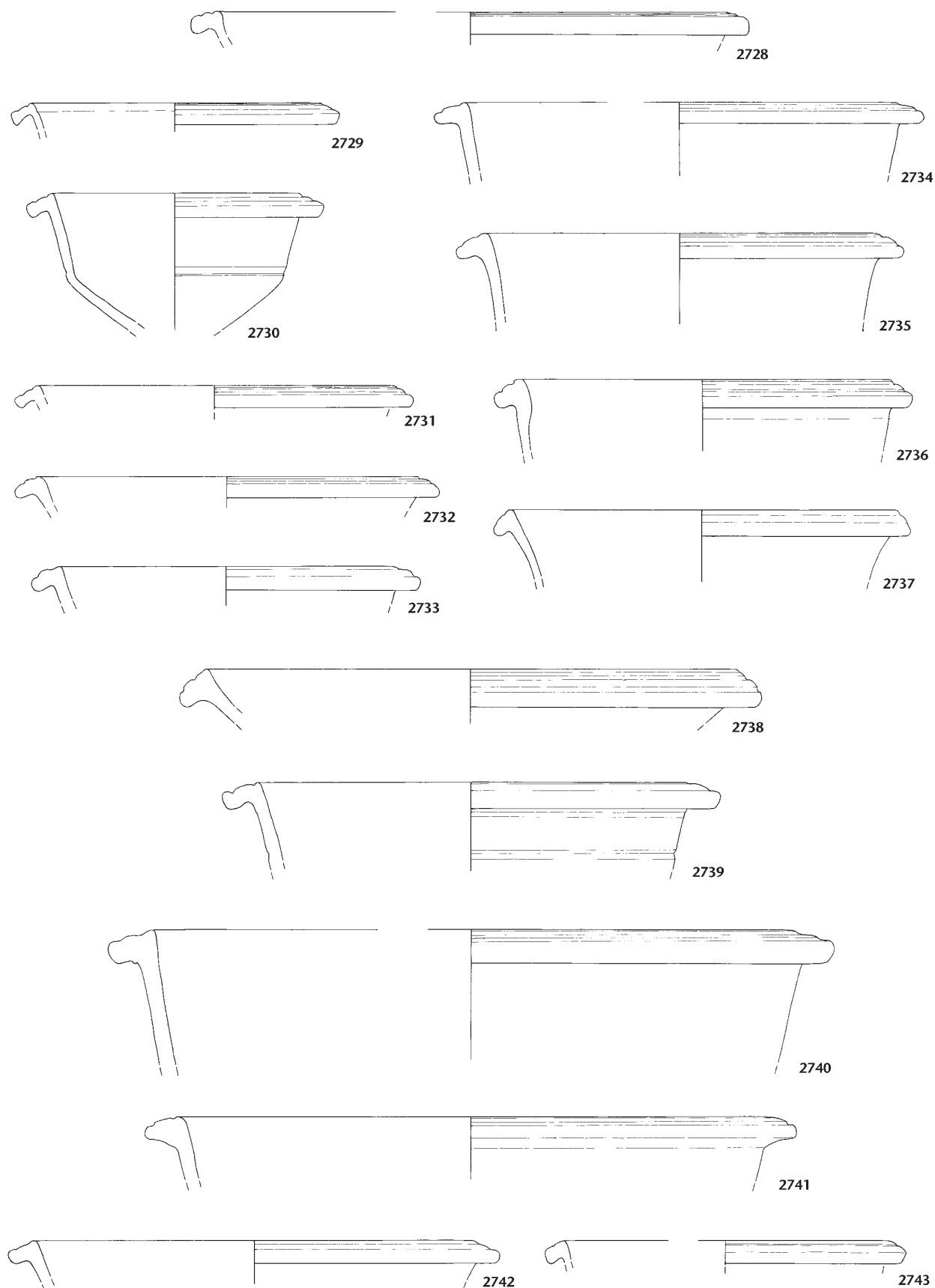
Tafel 133: Augst, Region 5,C: Schüsseln mit geradem bis leicht hängendem, gerilltem Horizontalrand ohne Überzug 2728–2743. M. 1:3.
